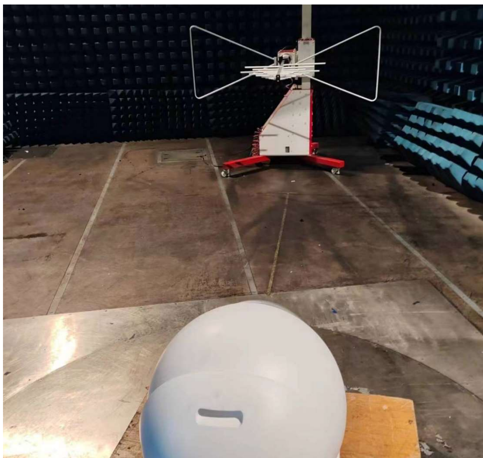
RE 30-1000MHz
