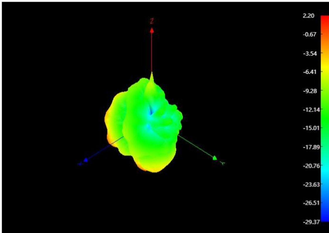
2400MHz 3D
