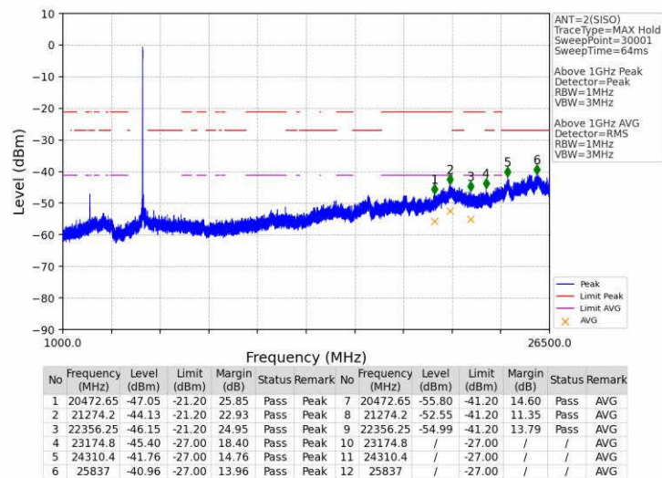
802.11a_LCH_5180MHz_Ant2_NTNV
