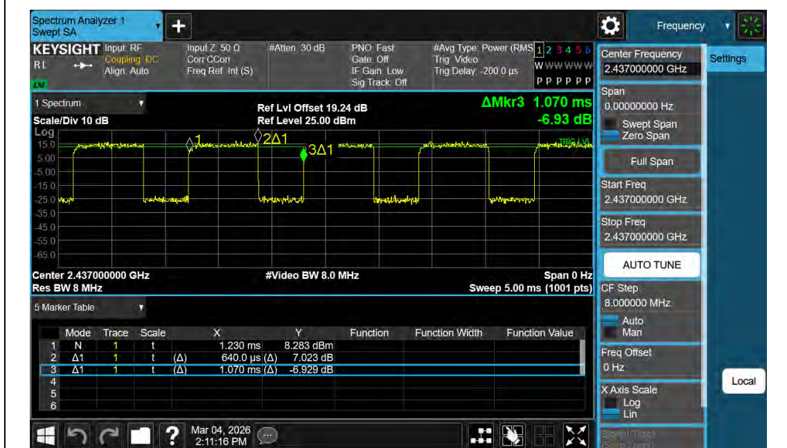
NTNV-11AX20MIMO-Ant1-2437
