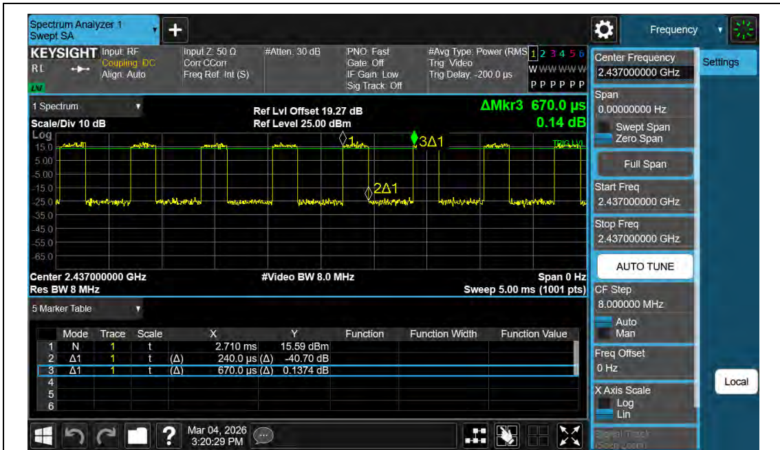
NTNV-11BE20MIMO-Ant2-2437
