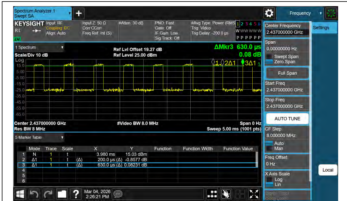
NTNV-11AX20MIMO-Ant2-2437
