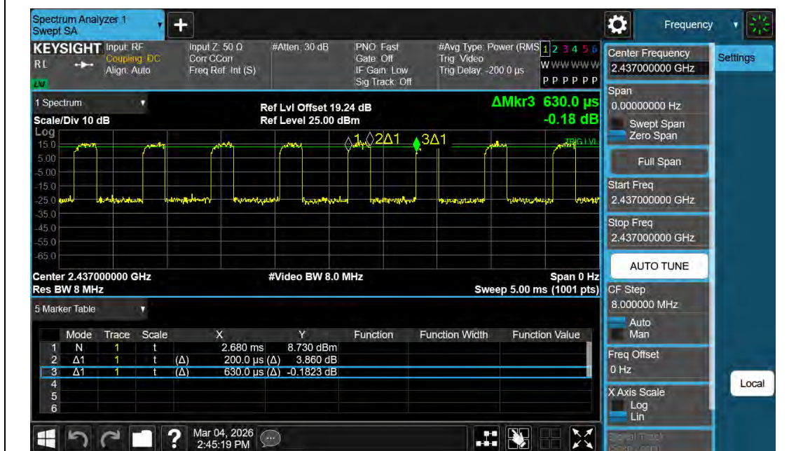
NTNV-11BE20MIMO-Ant1-2437
