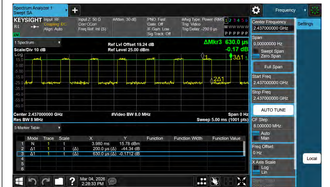
NTNV-11AX40MIMO-Ant1-2437
