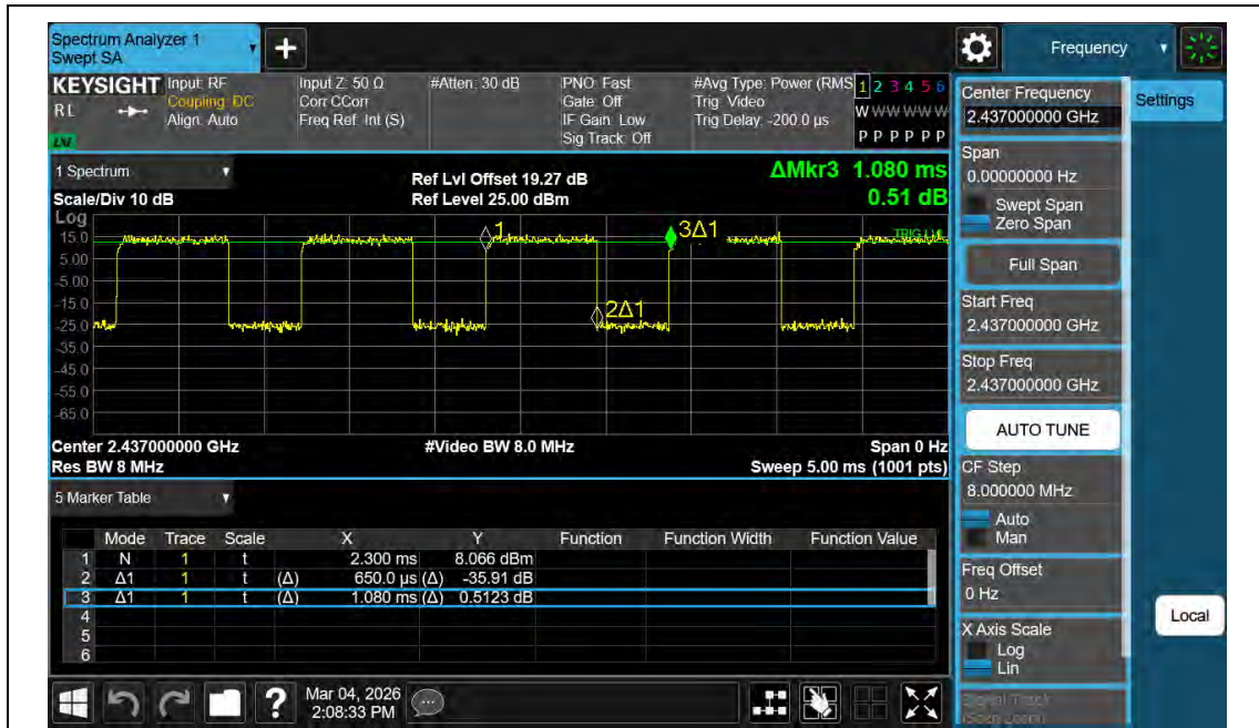
NTNV-11N40MIMO-Ant2-2437
