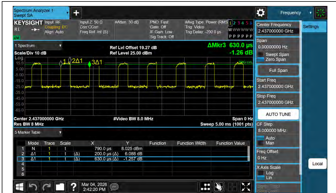
NTNV-11AX40MIMO-Ant2-2437
