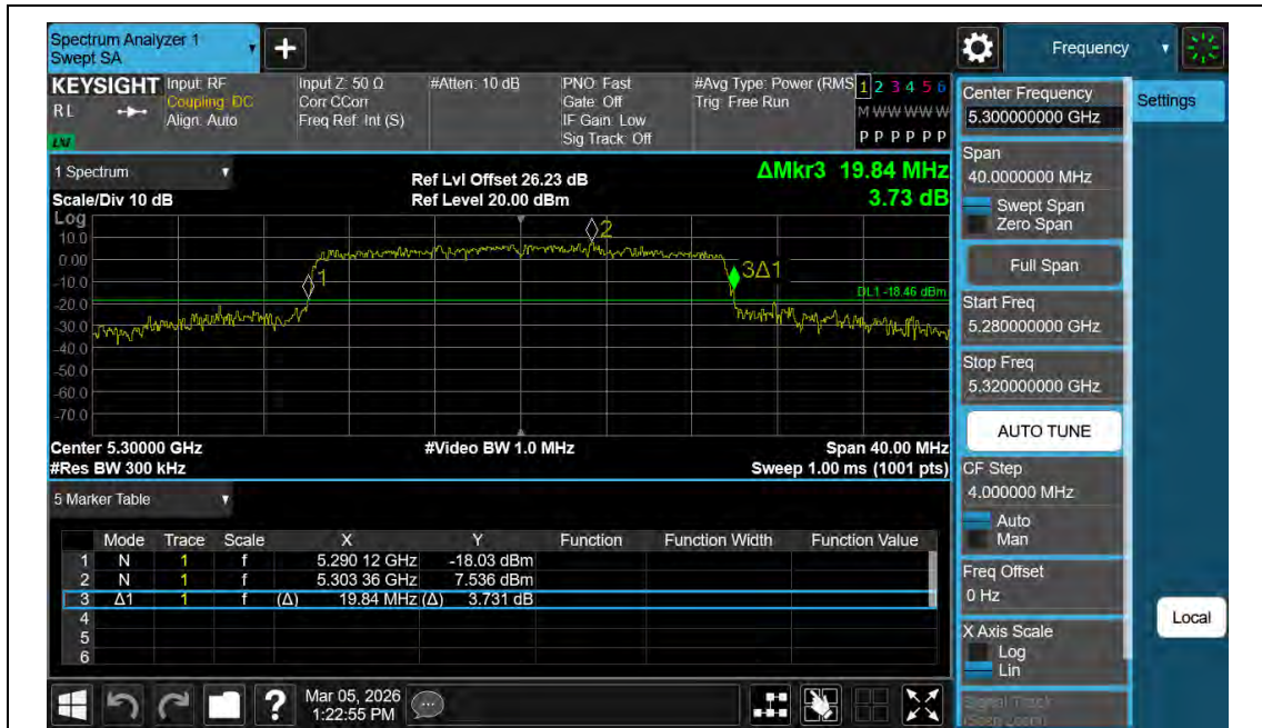
11AX20MIMO-Ant2-5300
