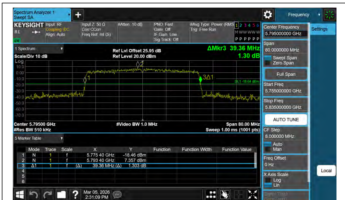
11AX40MIMO-Ant2-5795
