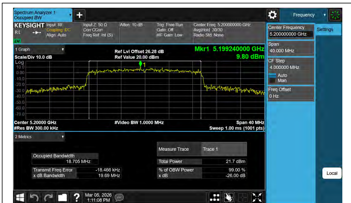
11AX20MIMO-Ant2-5200
