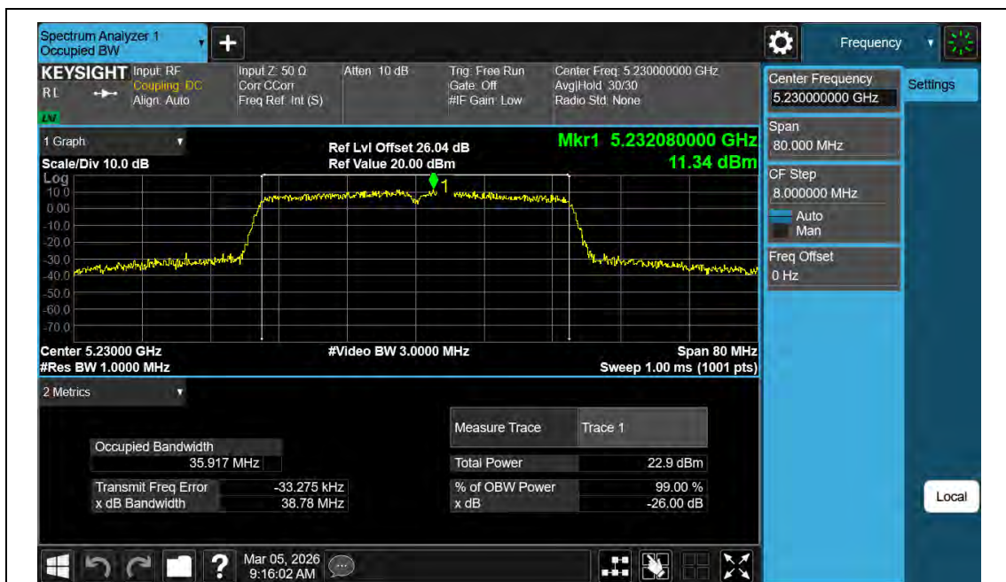
11N40MIMO-Ant2-5230
