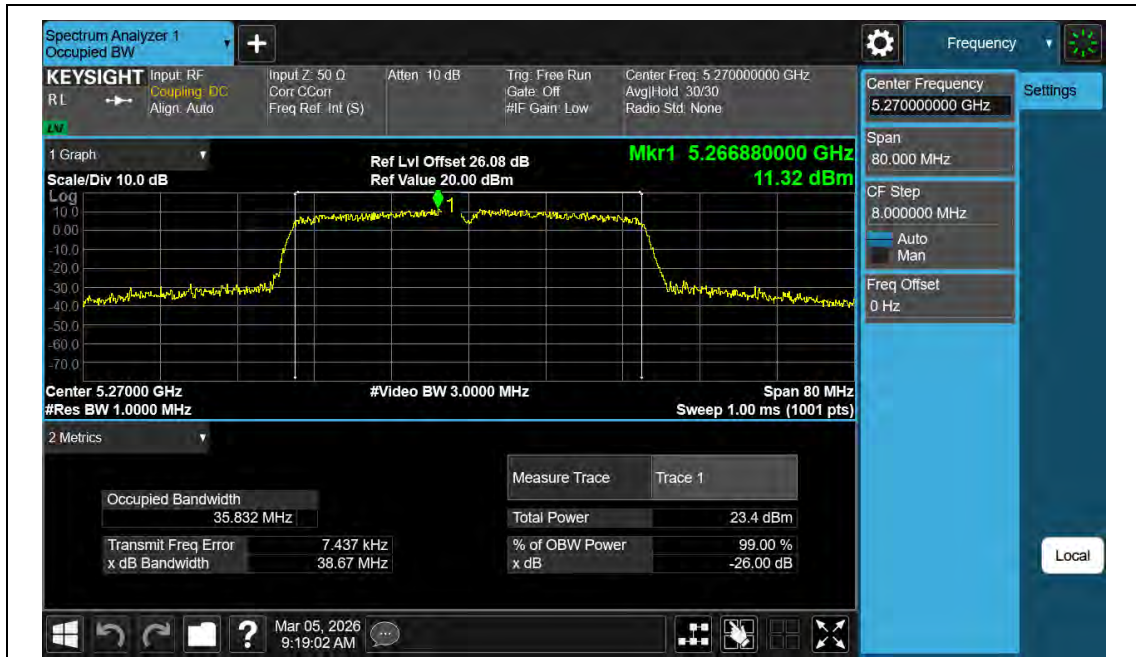
11N40MIMO-Ant2-5270
