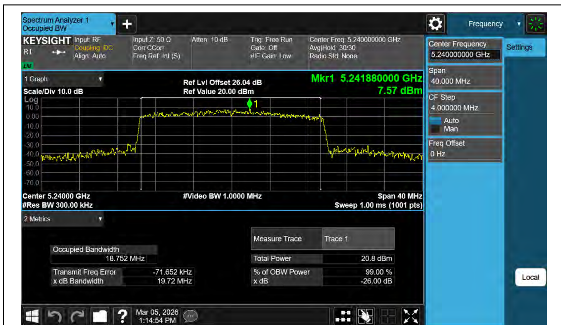
11AX20MIMO-Ant2-5240
