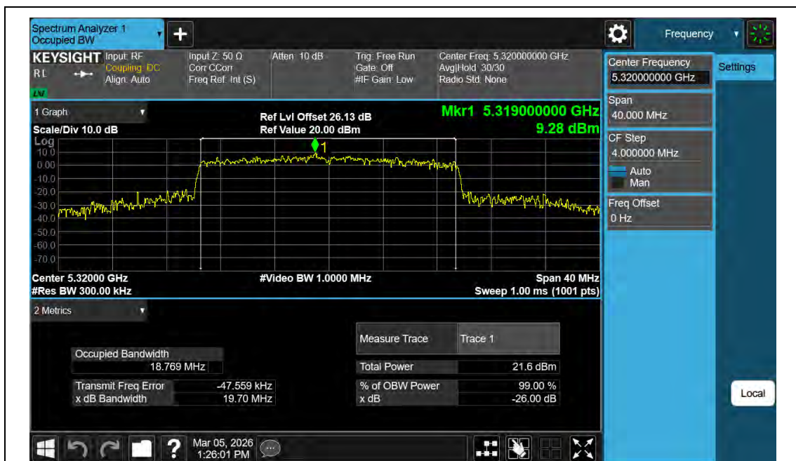
11AX20MIMO-Ant2-5320
