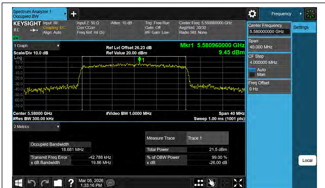
11AX20MIMO-Ant2-5580
