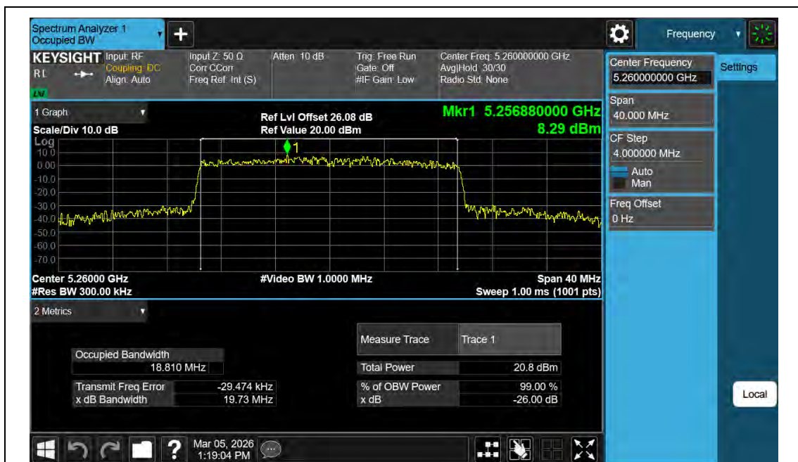
11AX20MIMO-Ant2-5260
