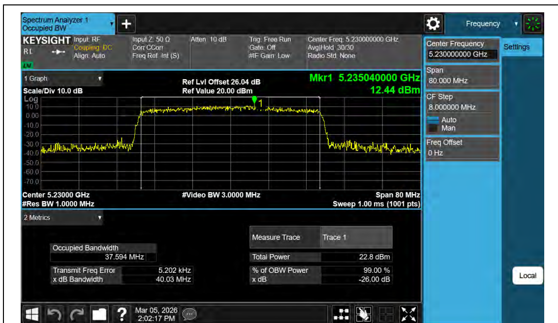
11AX40MIMO-Ant2-5230
