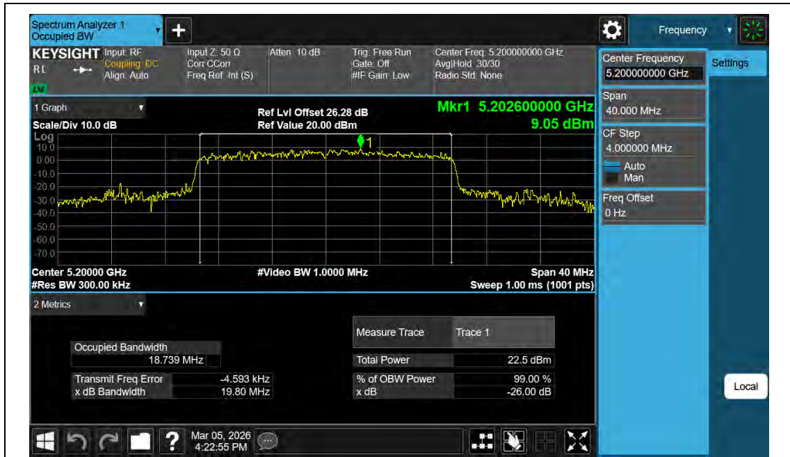
11BE20MIMO-Ant2-5200
