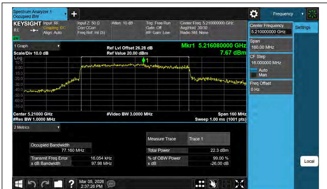
11AX80MIMO-Ant2-5210
