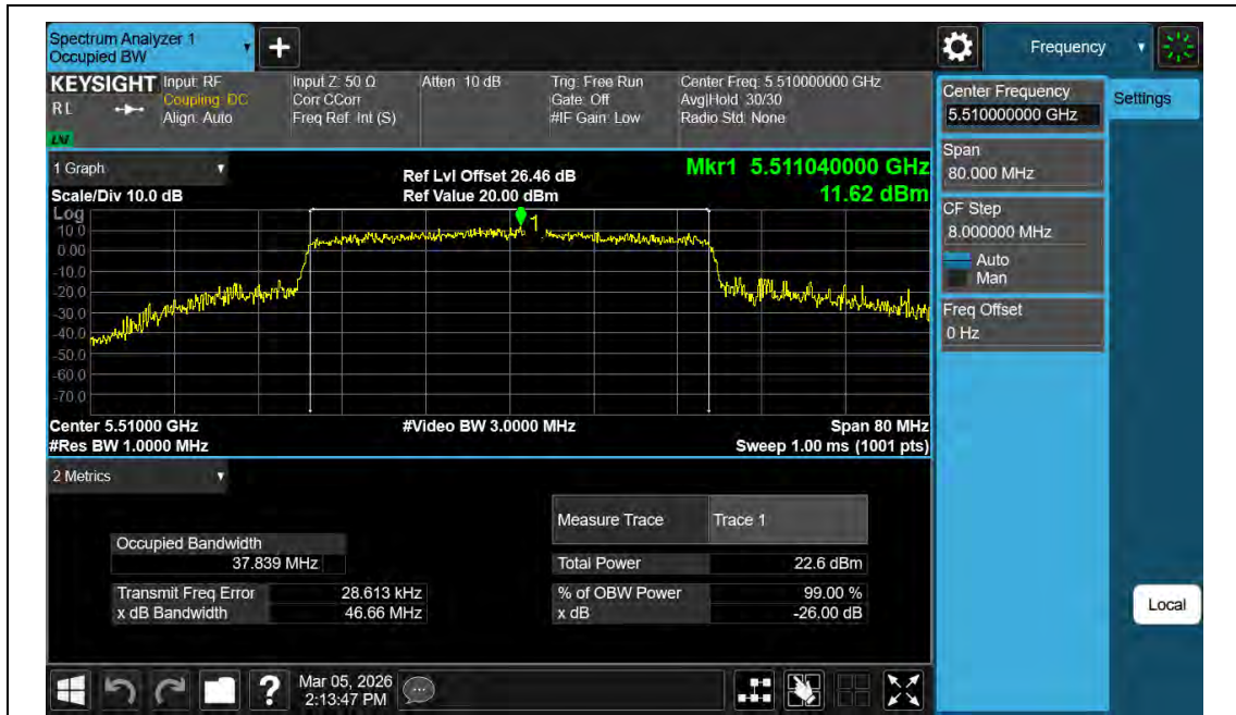
11AX40MIMO-Ant2-5510
