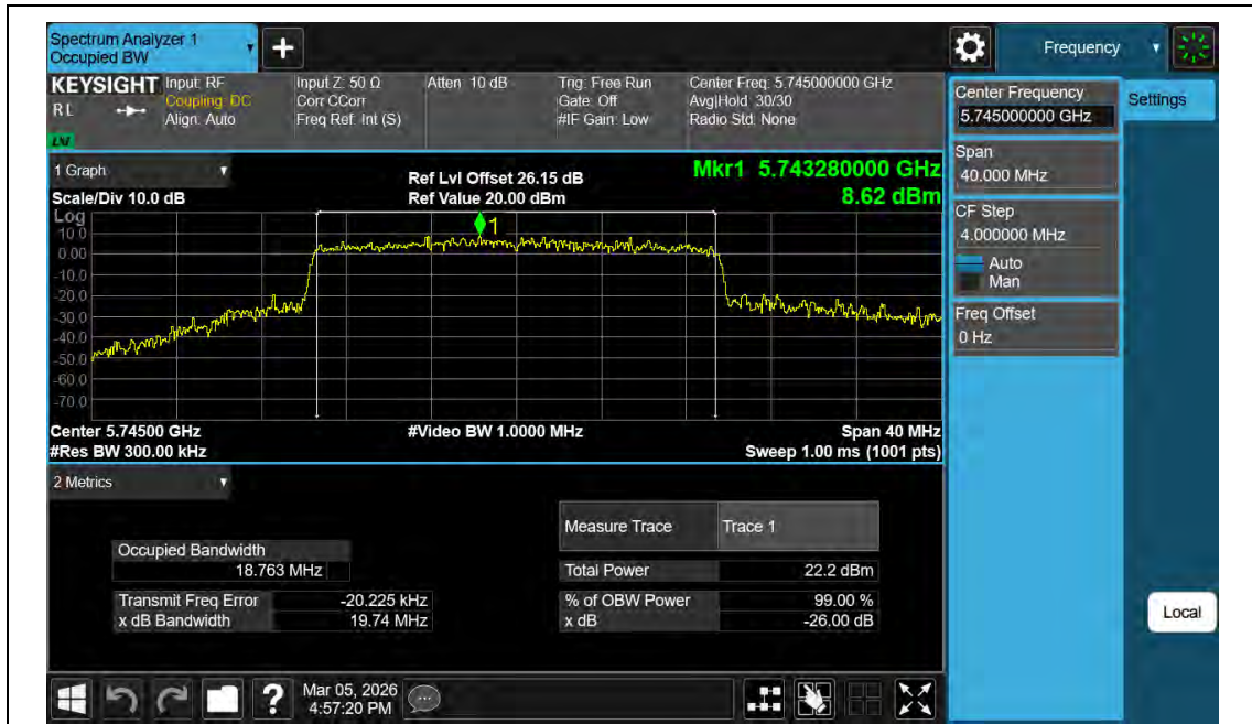
11BE20MIMO-Ant2-5745
