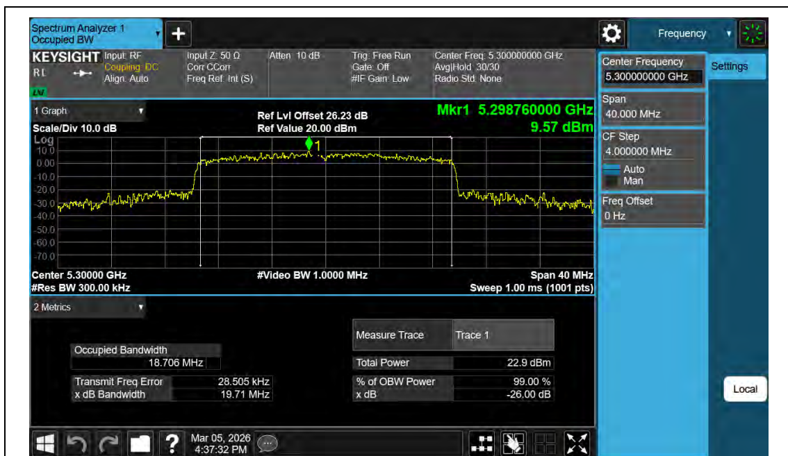
11BE20MIMO-Ant2-5300
