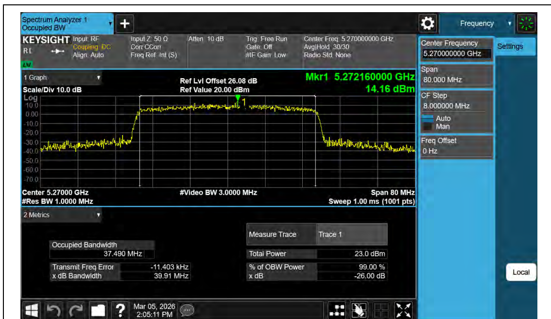
11AX40MIMO-Ant2-5270
