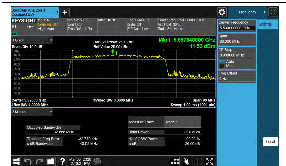
11AX40MIMO-Ant2-5590
