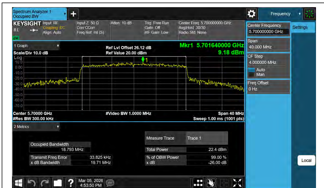
11BE20MIMO-Ant2-5700
