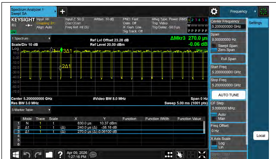
NTNV-11AX20MIMO-Ant2-5200
