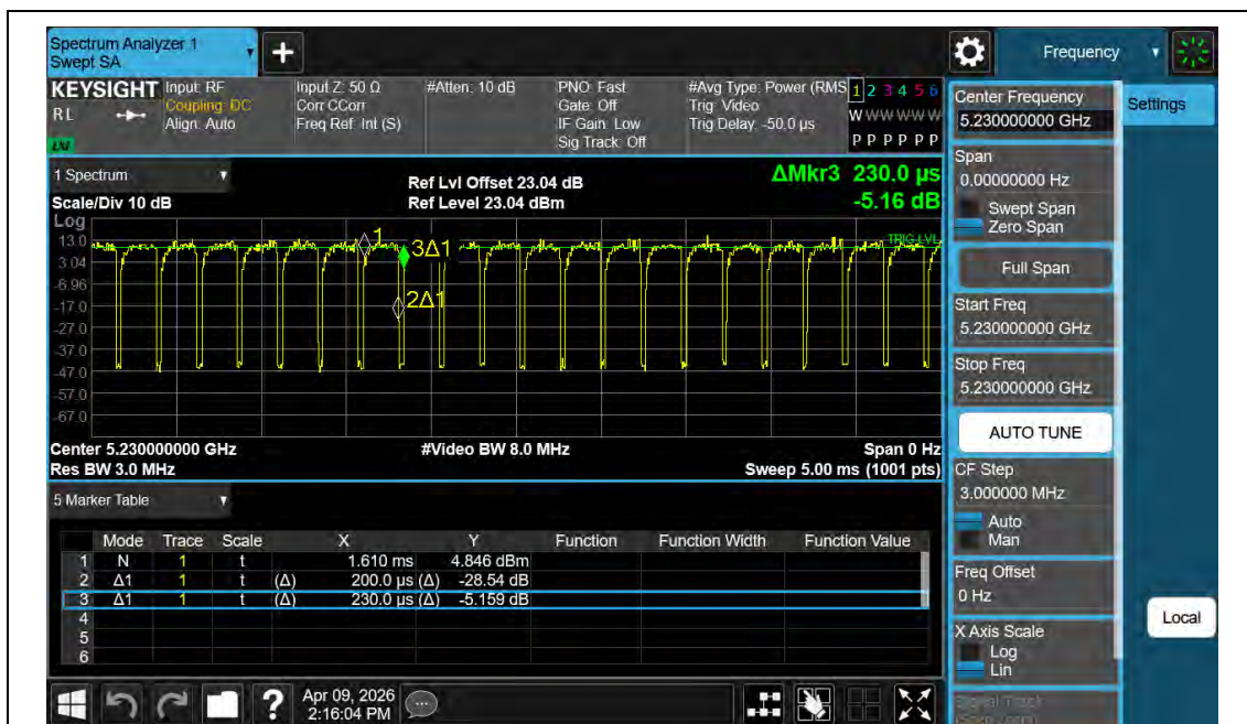
NTNV-11AX40MIMO-Ant2-5230
