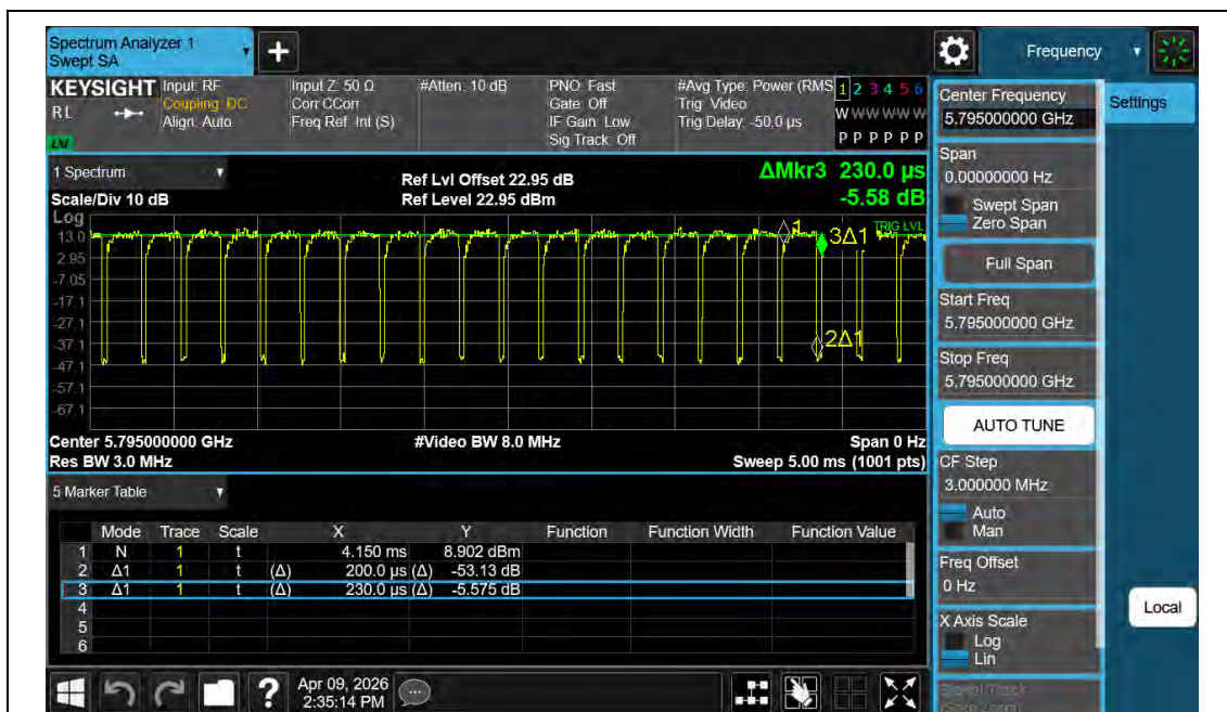
NTNV-11AX40MIMO-Ant2-5795
