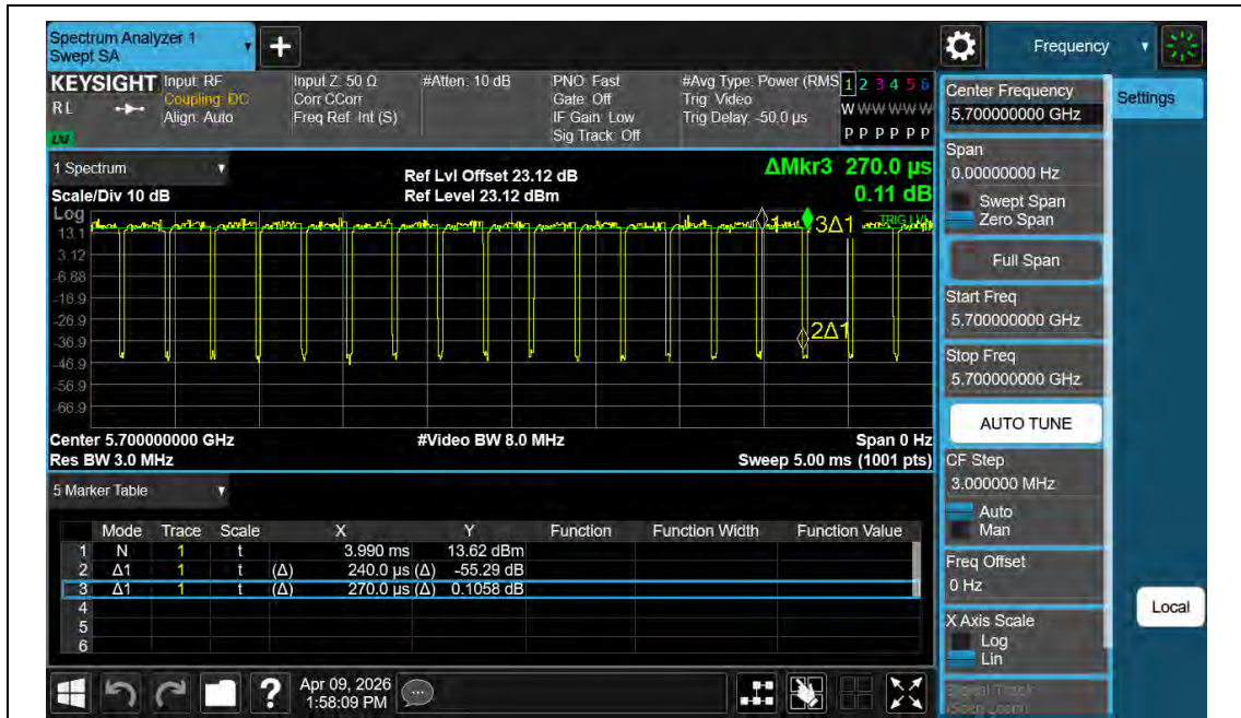
NTNV-11AX20MIMO-Ant2-5700
