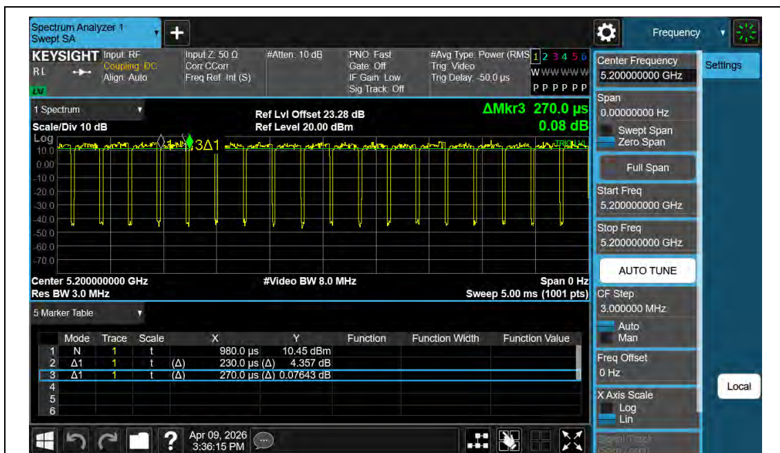
NTNV-11BE20MIMO-Ant2-5200
