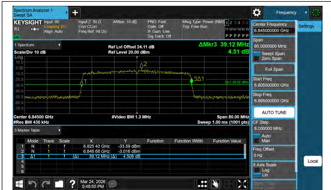
11AX40MIMO-Ant2-6845
