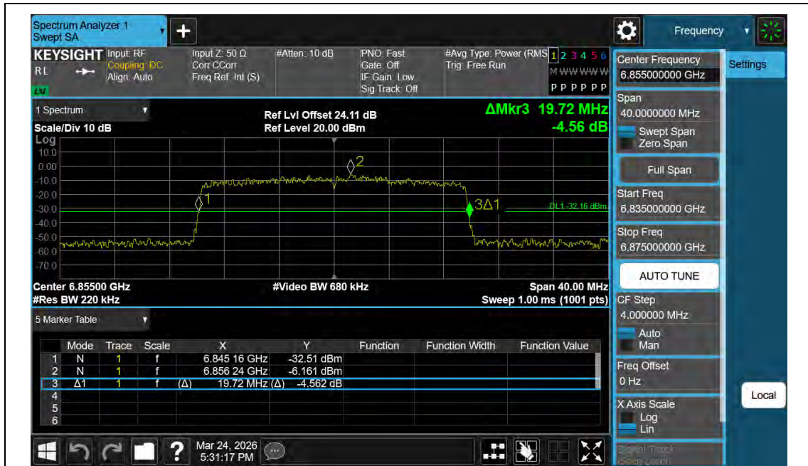
11AX20MIMO-Ant2-6855
