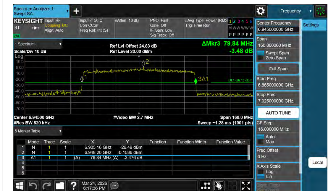
11AX80MIMO-Ant1-7025
