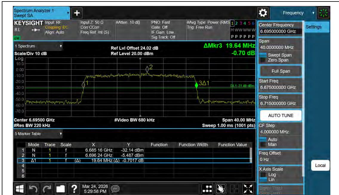
11AX20MIMO-Ant2-6695
