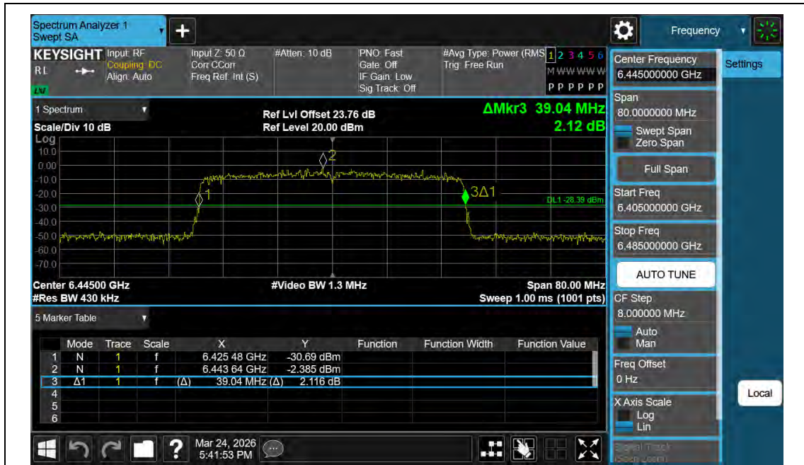
11AX40MIMO-Ant2-6445
