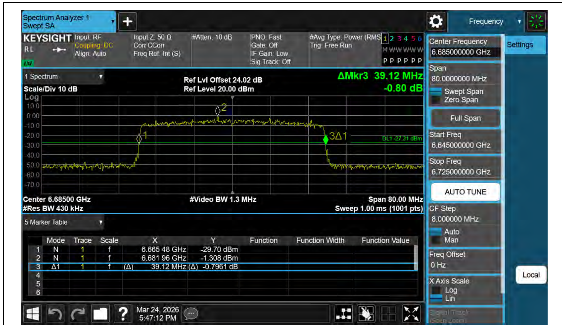
11AX40MIMO-Ant2-6685
