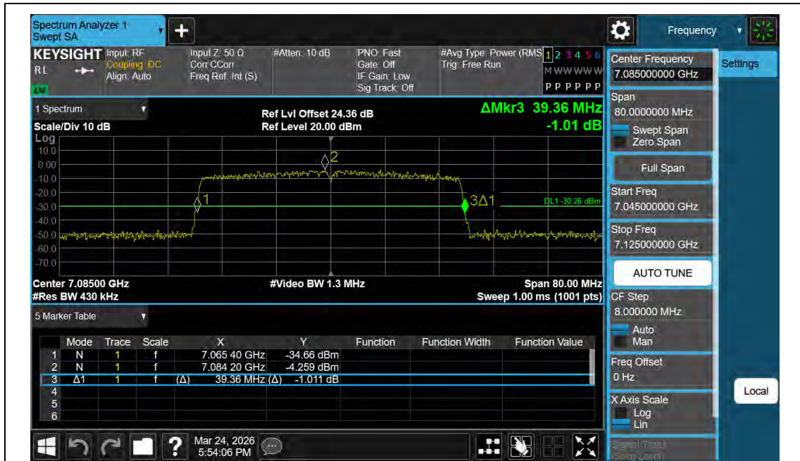
11AX40MIMO-Ant2-7085
