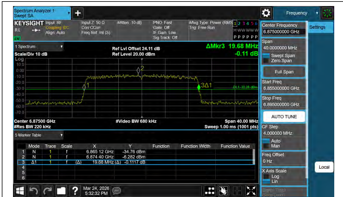
11AX20MIMO-Ant2-6875
