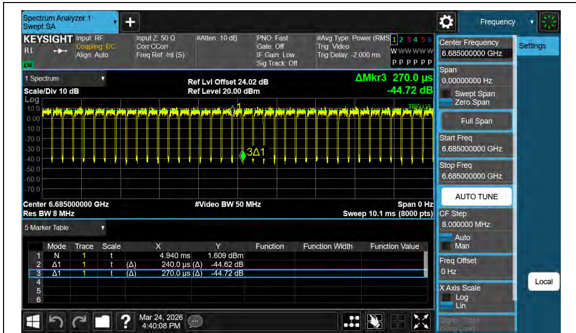
NTNV-11AX40MIMO-Ant2-6685
