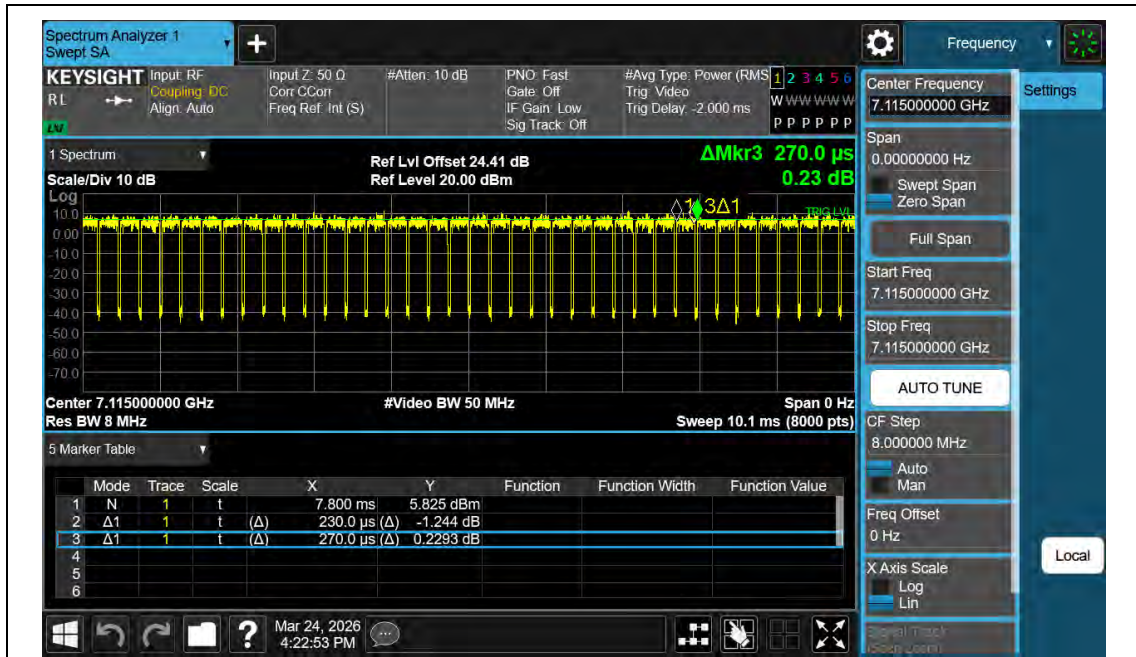
NTNV-11AX20MIMO-Ant2-7115
