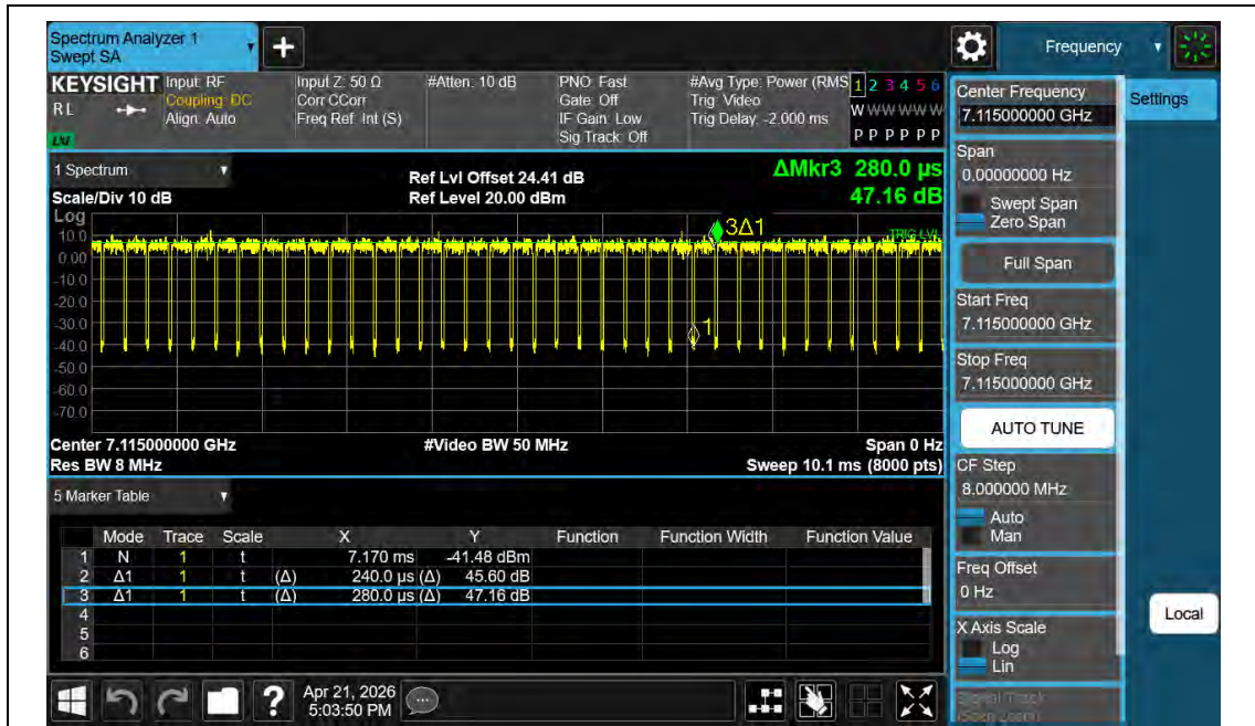
NTNV-11BE20MIMO-Ant2-7115
