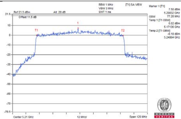
802.11ax (HE80)_Full RU / Chain 1 / CH 42
