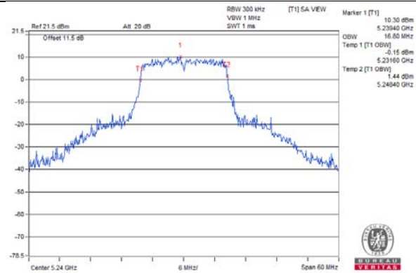
802.11ax (HE20)_Full RU / Chain 1 / CH 48
