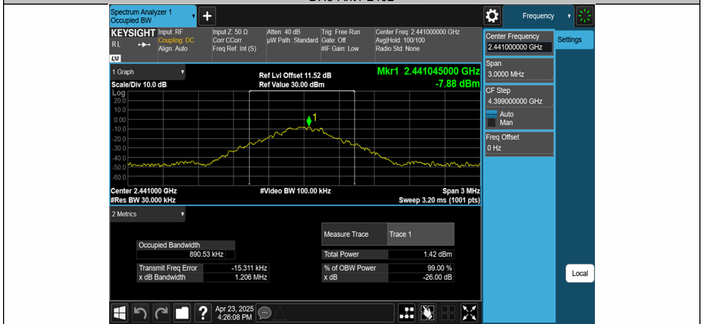
DH5-Ant1-2441
