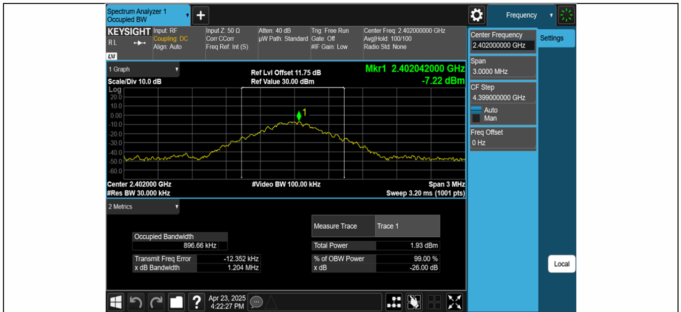
DH5-Ant1-2402
