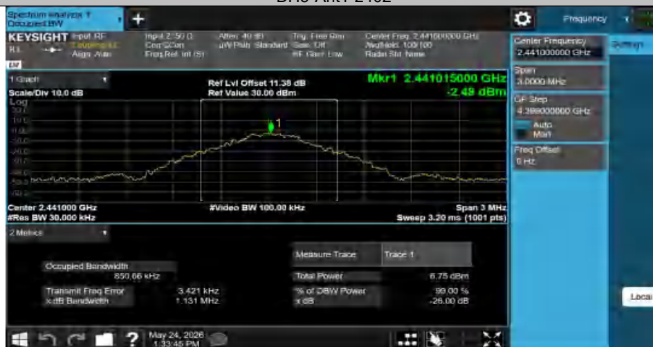
DH5-Ant1-2441
