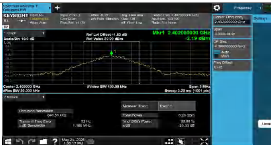
DH5-Ant1-2402
