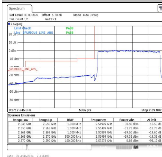
Band38_20MHz_QPSK_37850_100RB#0
