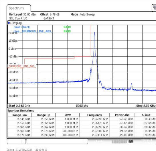
Band38_20MHz_QPSK_37850_1RB#0
