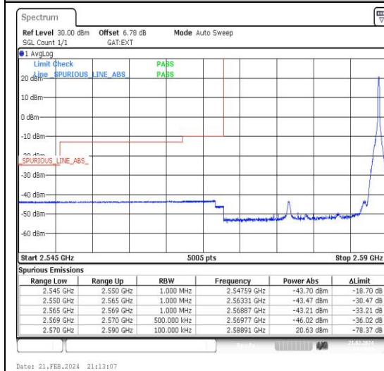
Band38_20MHz_QPSK_37850_1RB#99
