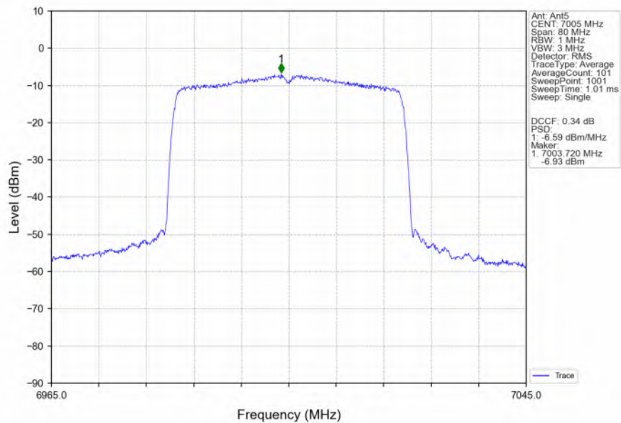
802.11ax(HEW40) MCH 7005MHz SU / Ant5 NTN
