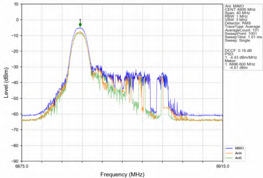
802.11ax(HEW20) LCH 6895MHz RU26 Left MIMO NTN
