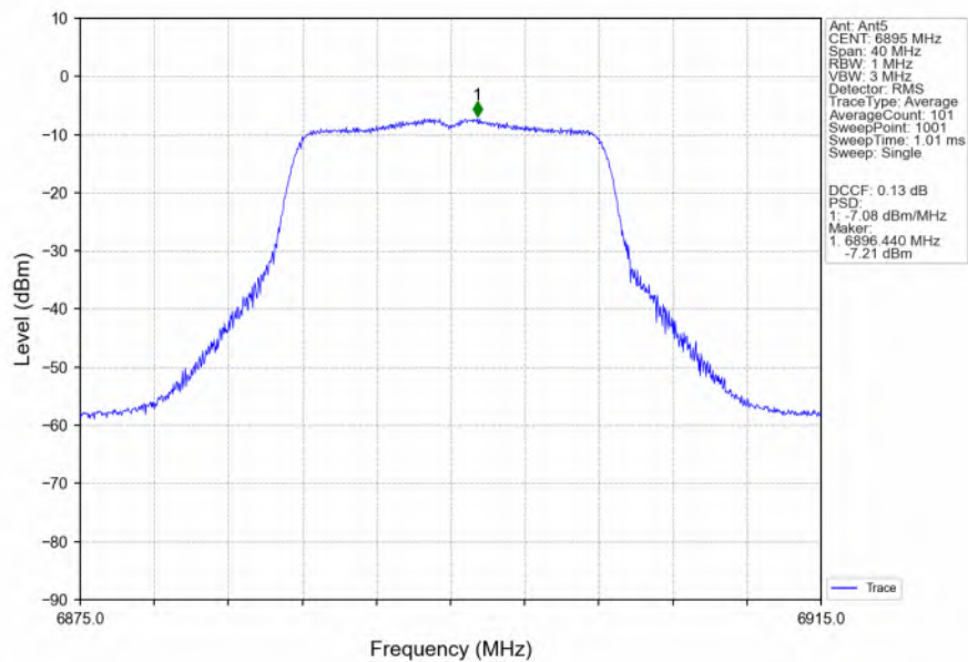
802.11a_LCH_6895MHz_Ant5_NTNV
