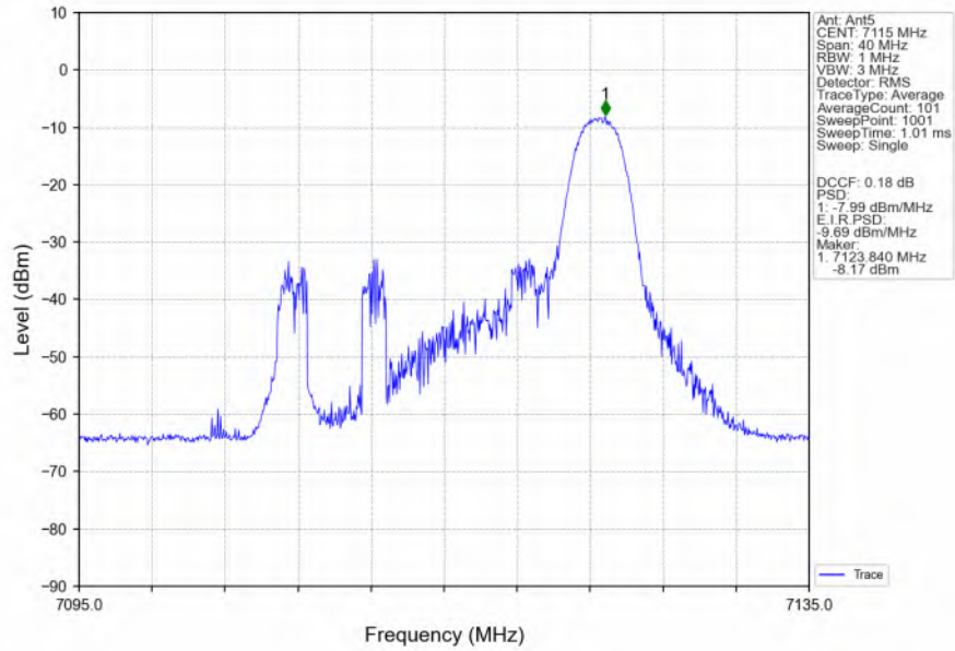
802.11ax(HEW20) HCH 7115MHz RU26 Left MIMO_NTNV
