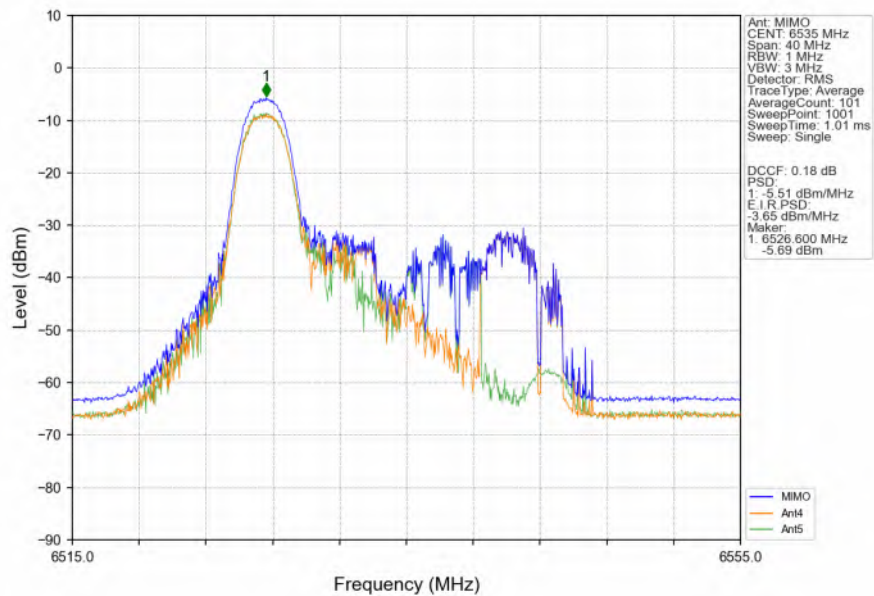
802.11ax(HEW20) LCH 6535MHz RU26 Left MIMO NTN
