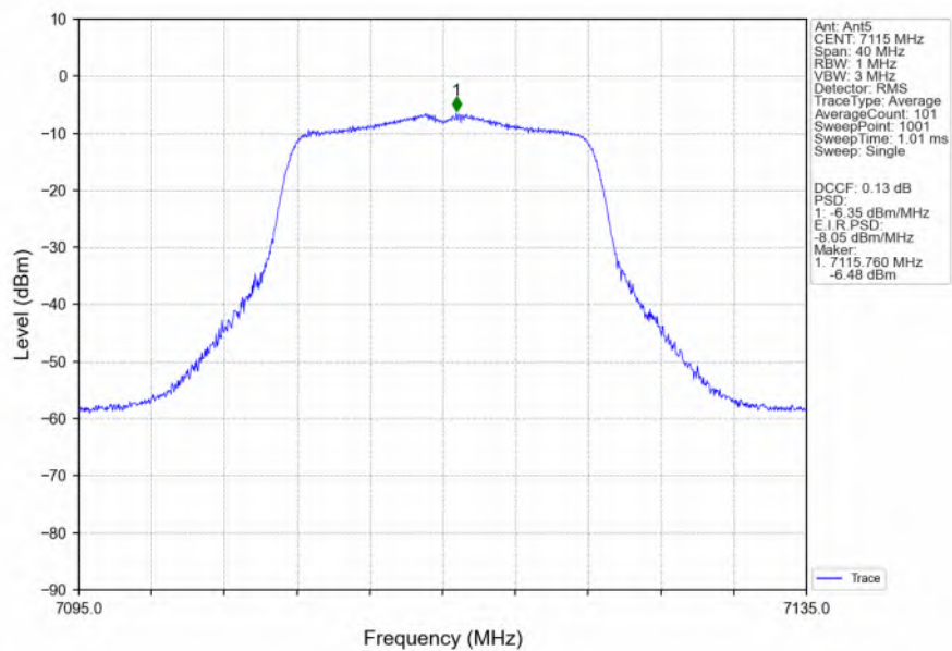
802.11a_HCH_7115MHz_Ant5_NTNV
