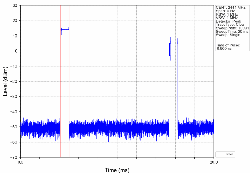
Pi/4DQPSK_2DH1_HOPP_Ant4_NTNV
