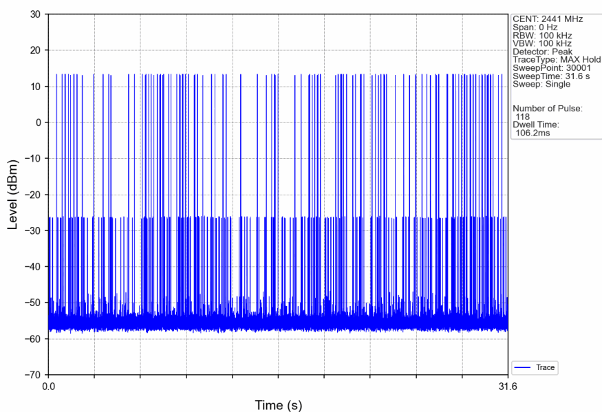
Pi/4DQPSK_2DH1_HOPP_Ant4_NTNV
