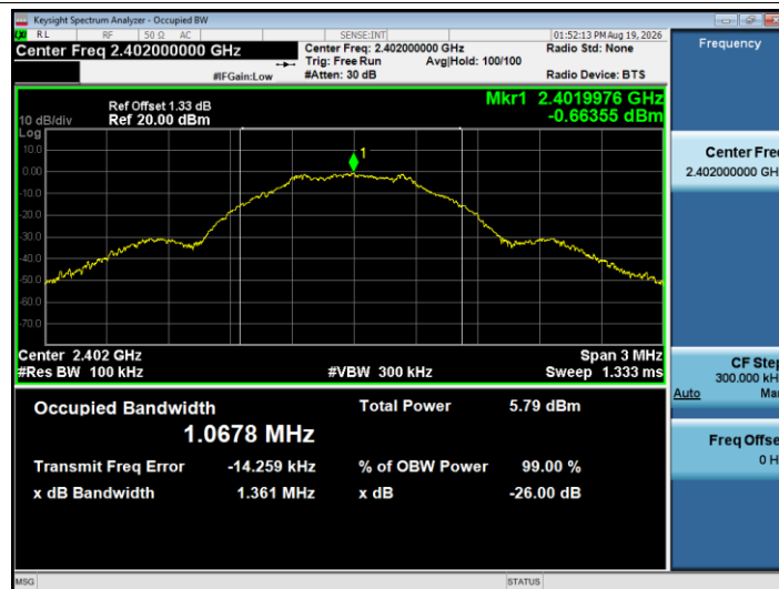
OBW NVNT BLE 1M 2402MHz Ant1
