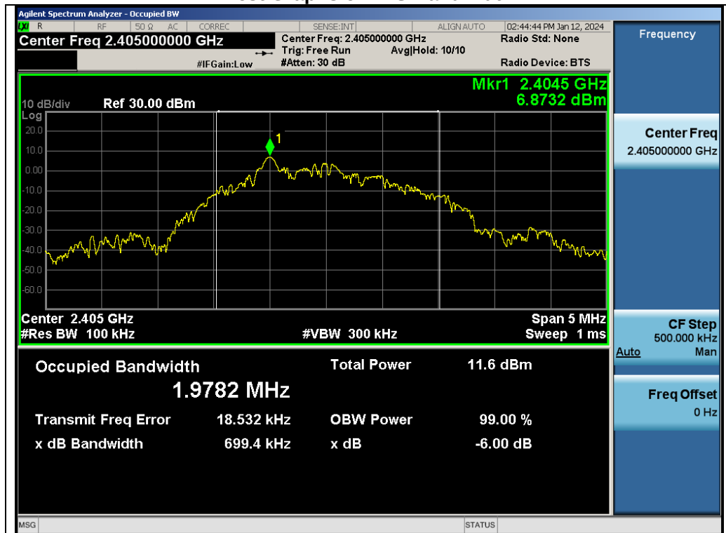
Test_Graph_ANT1_2405_DTSBW
