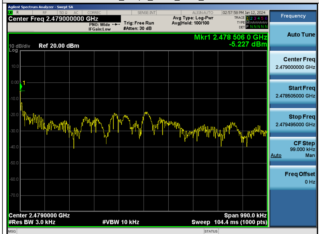
Test_Graph_ANT1_2479_PSD
