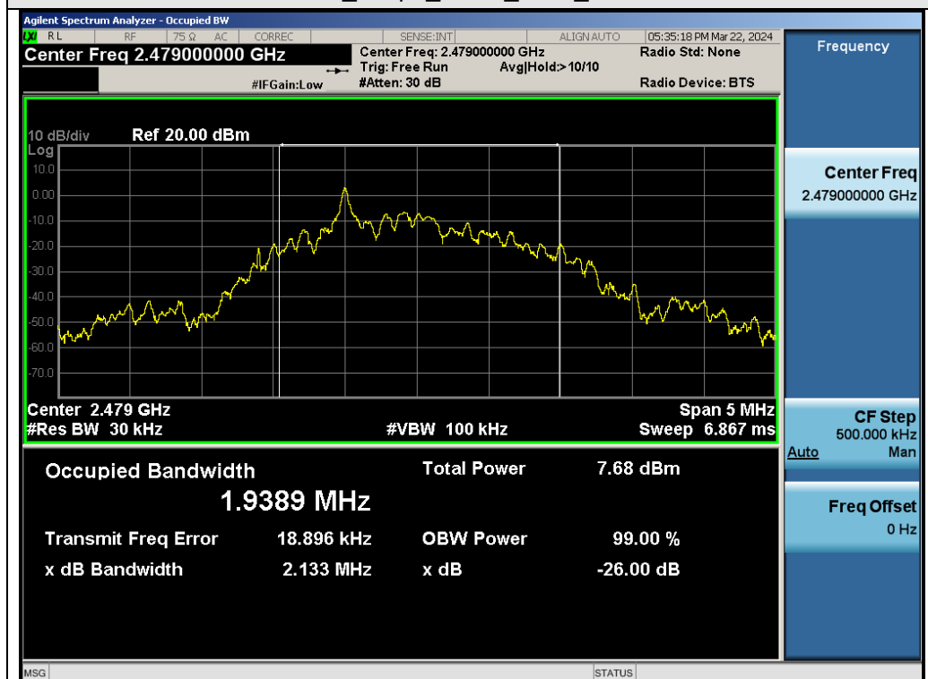
Test_Graph_ANT1_2479_OBW
