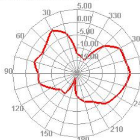
5421.426MHz E1
