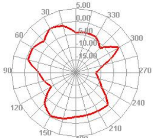
5635.710MHz H
