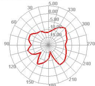
5421.426MHz E2
