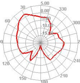
849.994MHz E1
