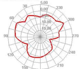
5849.994MHz H
