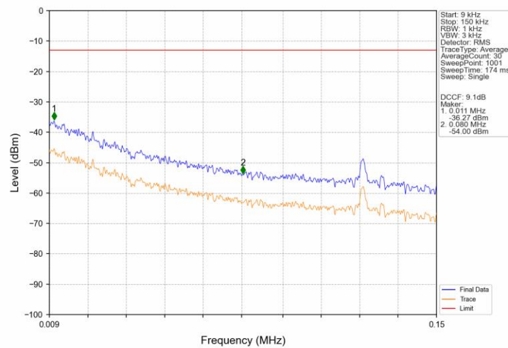
GSM850_GSM_LCH_824.2MHz_GSM_NTNV
