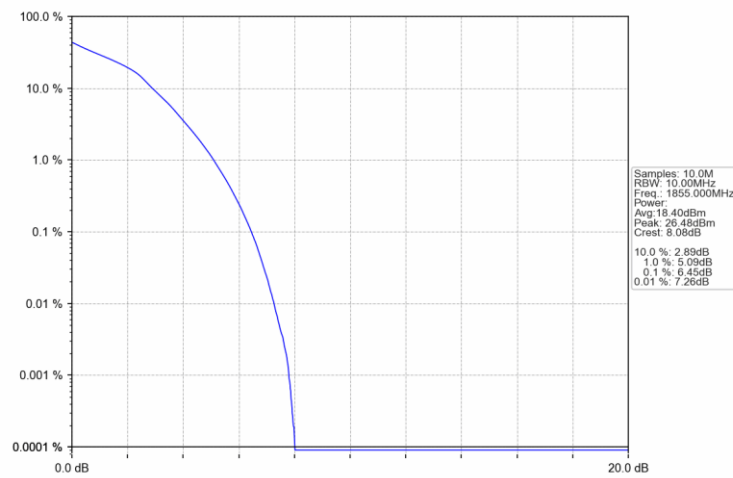
Band2_10MHz_16QAM_LCH_1855MHz_RB_50_0_NTNV
