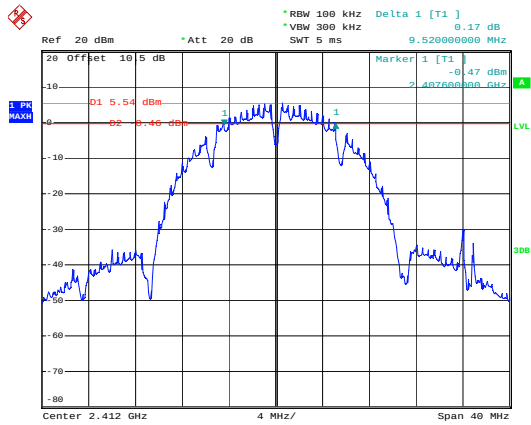
b_2412MHz_Chain 0
