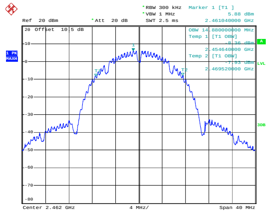
b_2462MHz_Chain 0
