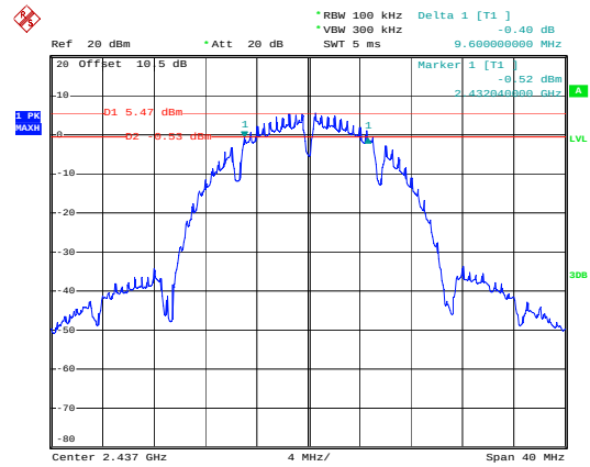
b_2437MHz_Chain 0
