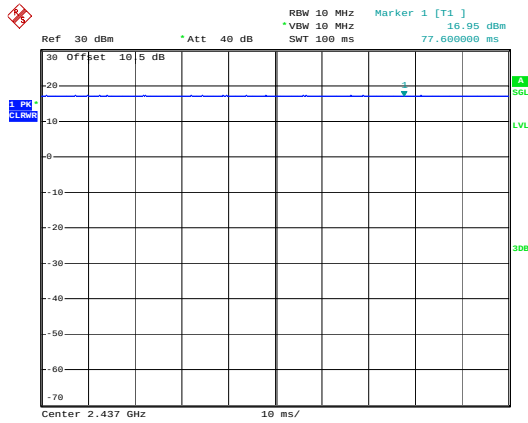
b_2437MHz_Chain 0
