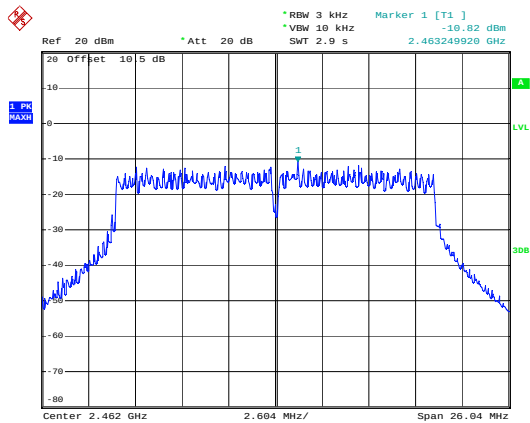
n20_2462MHz_Chain 0
