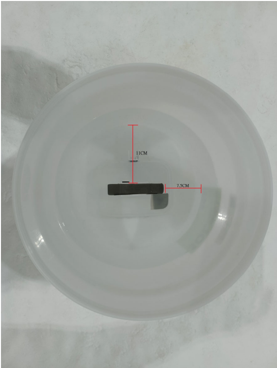
DUT Position
