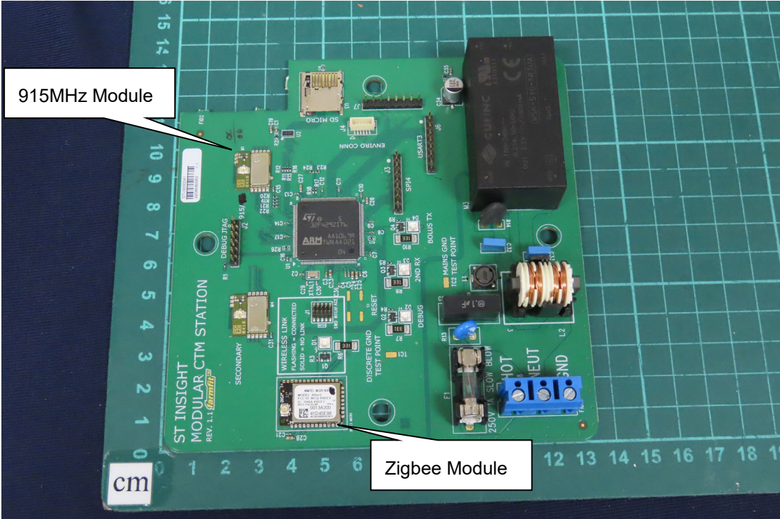
(13)EUT Photo
