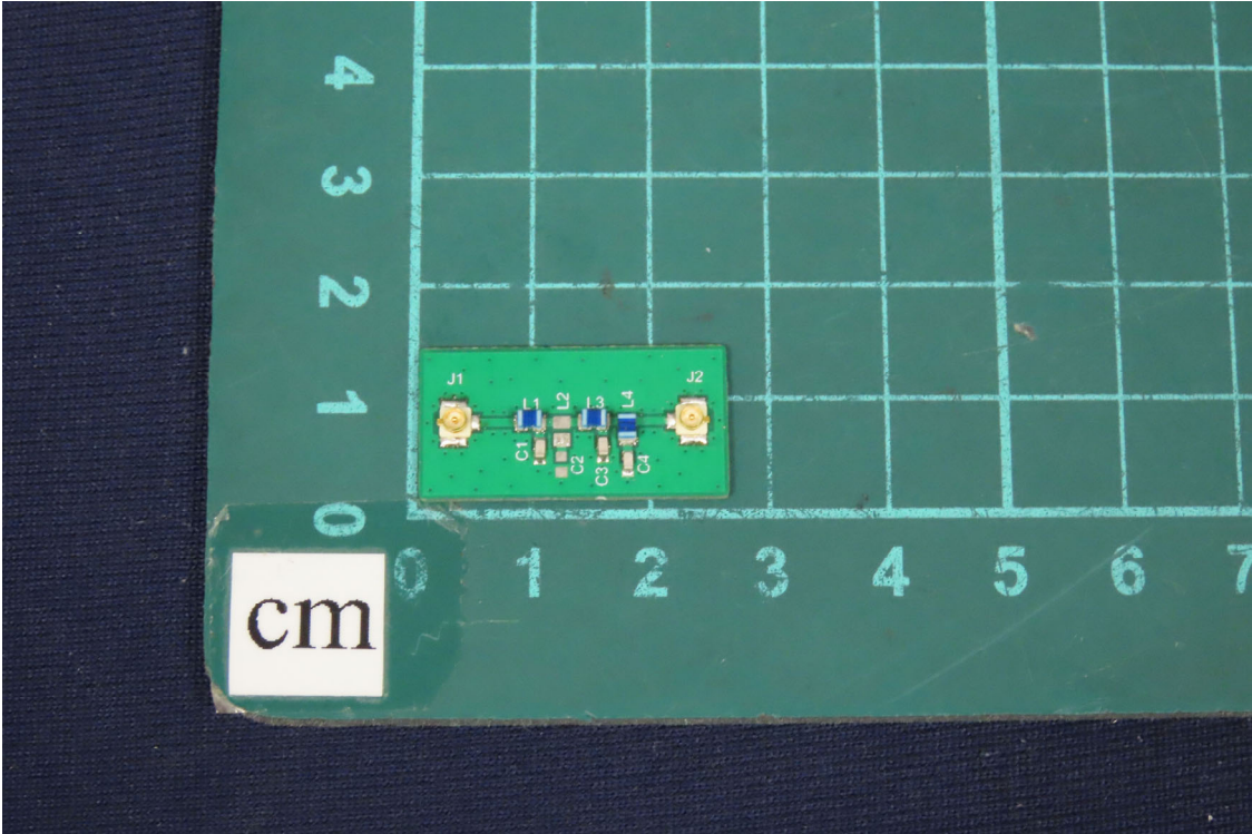
(10)EUT Photo
