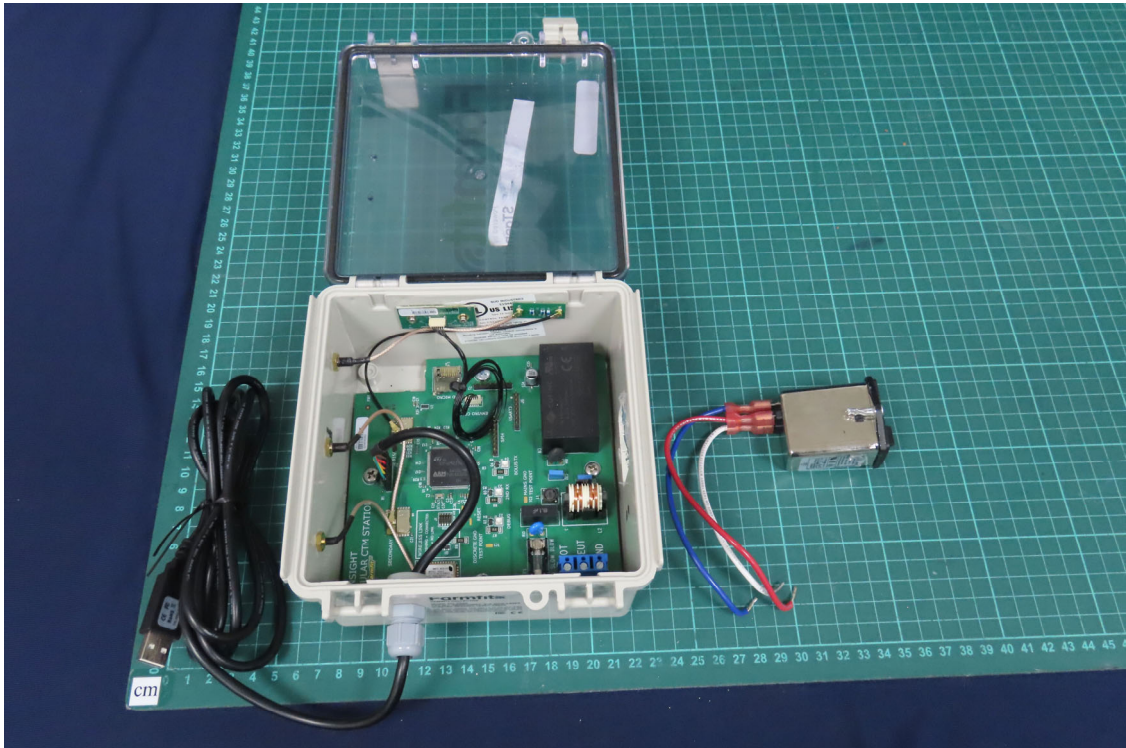
(8) EUT Photo
