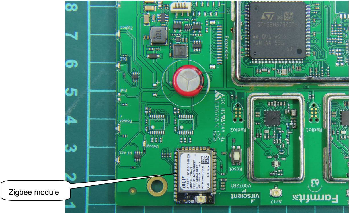
(40) EUT Photo
