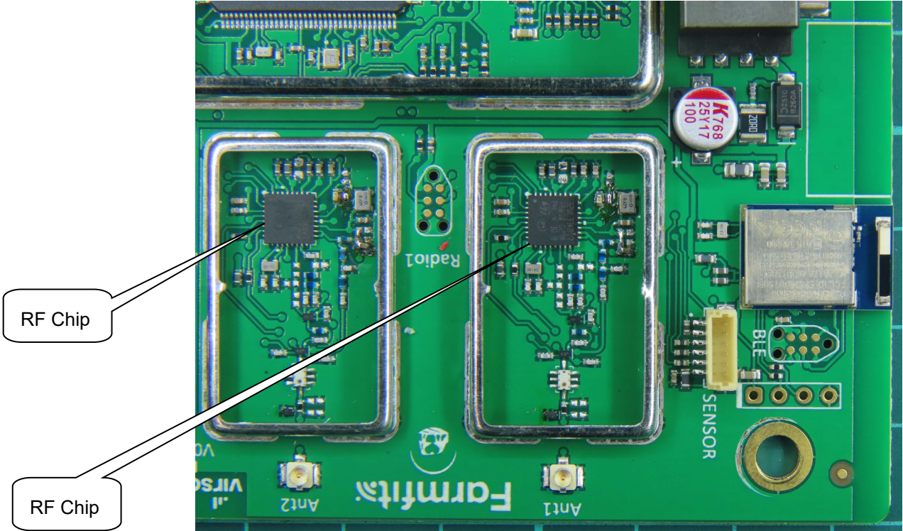
(31) EUT Photo
