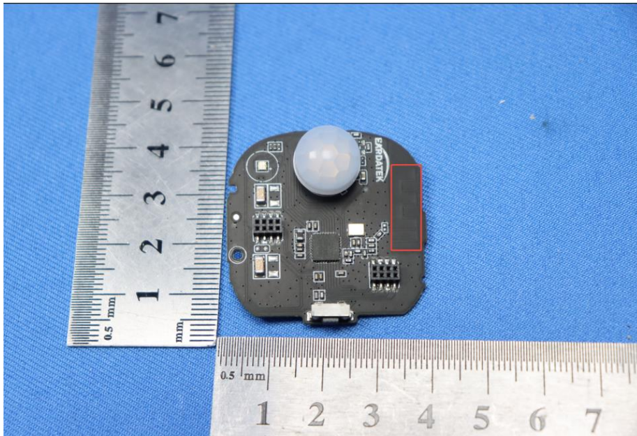
BLE Antenna Location
