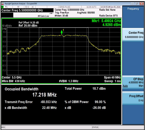
11A-Ant1-5500
