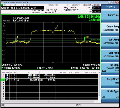
11N40SISO-Ant1-5270
