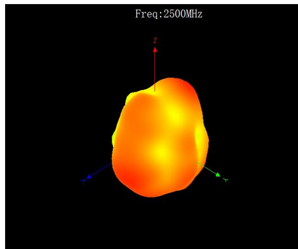
2500MHz 3D
