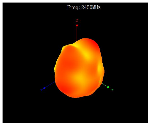
2450MHz 3D
