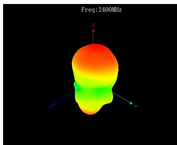
2400MHz 3D 放类似图 Z 轴朝上
