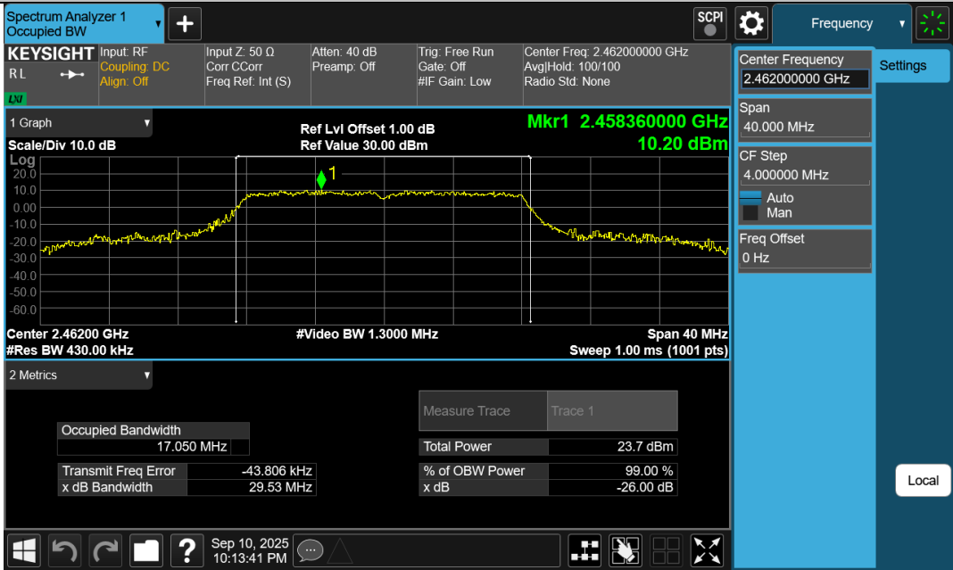
11G-Ant1-2462
