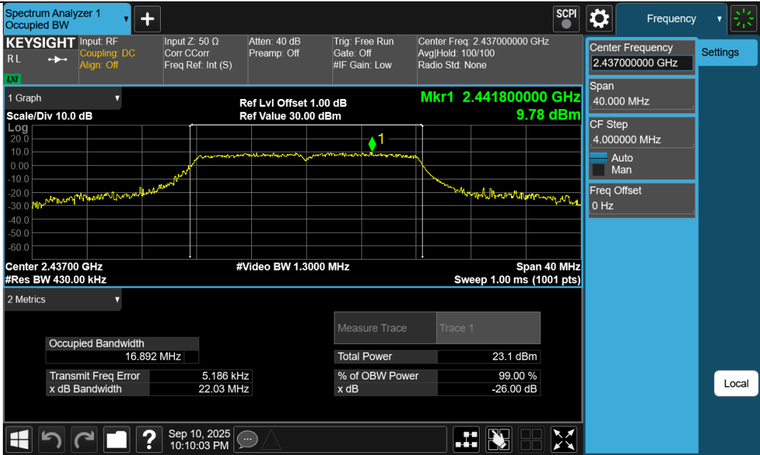
11G-Ant1-2437
