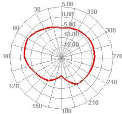
5850.000MHz H
