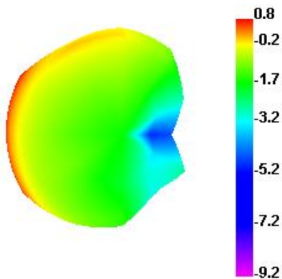
5150.000MHz E1
