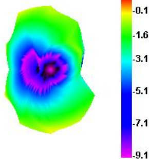
2450.000MHz E1
