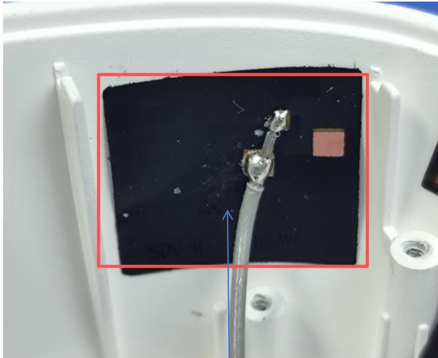
Antenna
