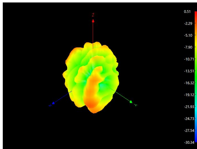
5450MHz 3D
