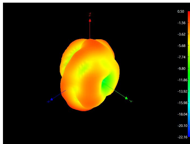
2450MHz 3D
