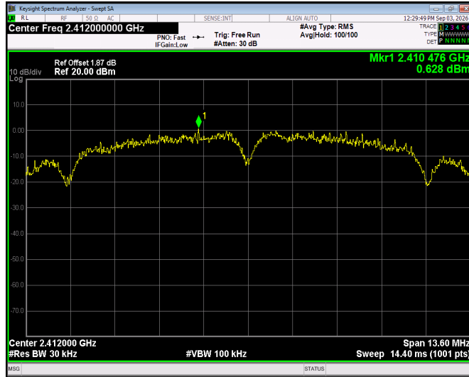
802.11b - CH01
