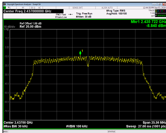
802.11n20 - CH06
