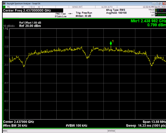
802.11b - CH06
