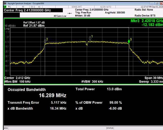
802.11g - CH01
