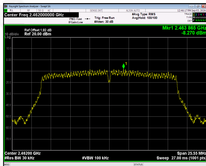
802.11n20 - CH11
