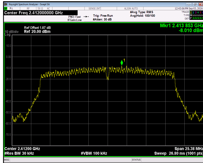
802.11n20 - CH01
