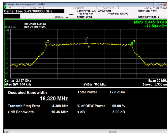
802.11g - CH06
