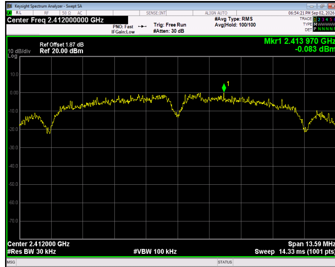
802.11b - CH01
