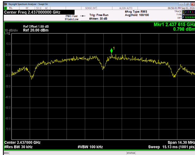
802.11b - CH06
