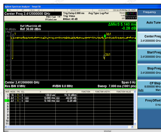
802.11n(H20)
