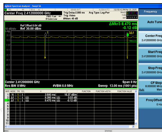
802.11b
