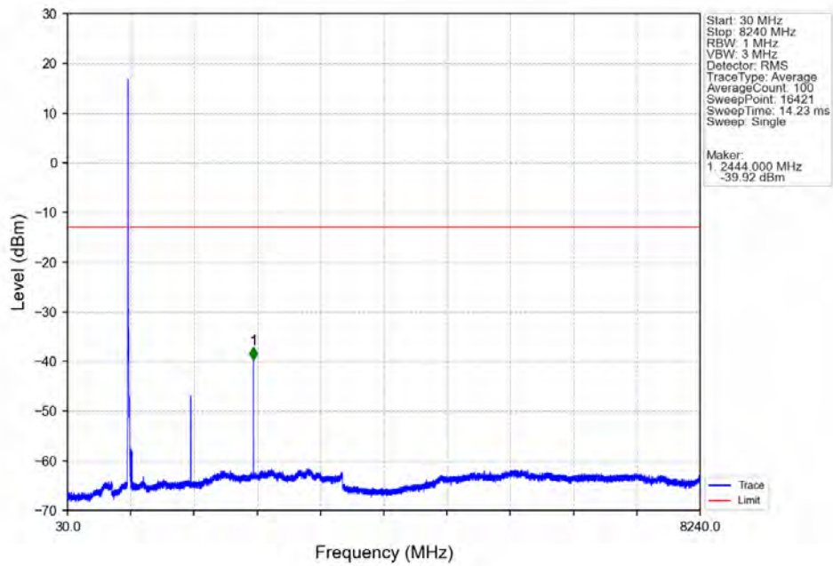
Band26a 10MHz 256QAM LCH 819MHz RB 50 0 NTNV
