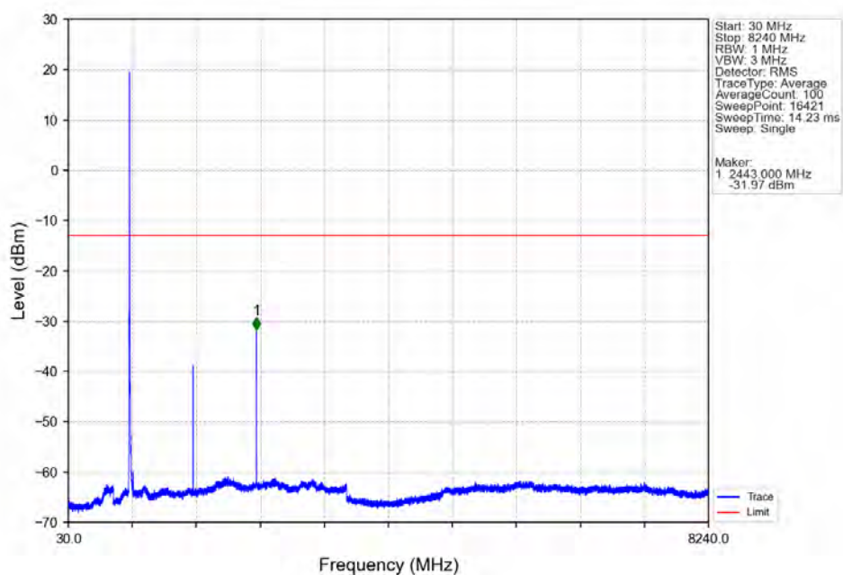
Band26a 5MHz 64QAM LCH 816.5MHz RB 1 0 NTNV
