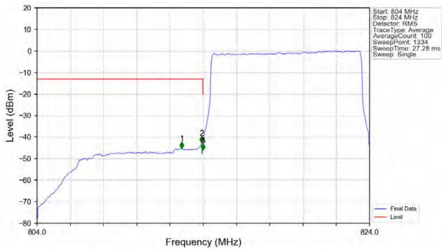
Band26a 10MHz 256QAM LCH 819MHz RB 50 0 NTNV
