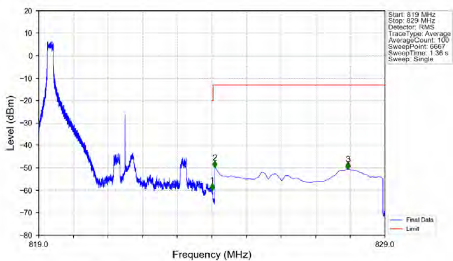
Band26a 5MHz 64QAM HCH 821.5MHz RB 1 24 NTNV
