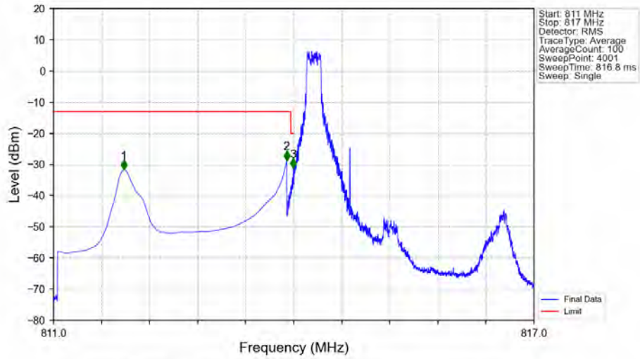
Band26a 1.4MHz 64QAM LCH 814.7MHz RB 1 0 NTNV
