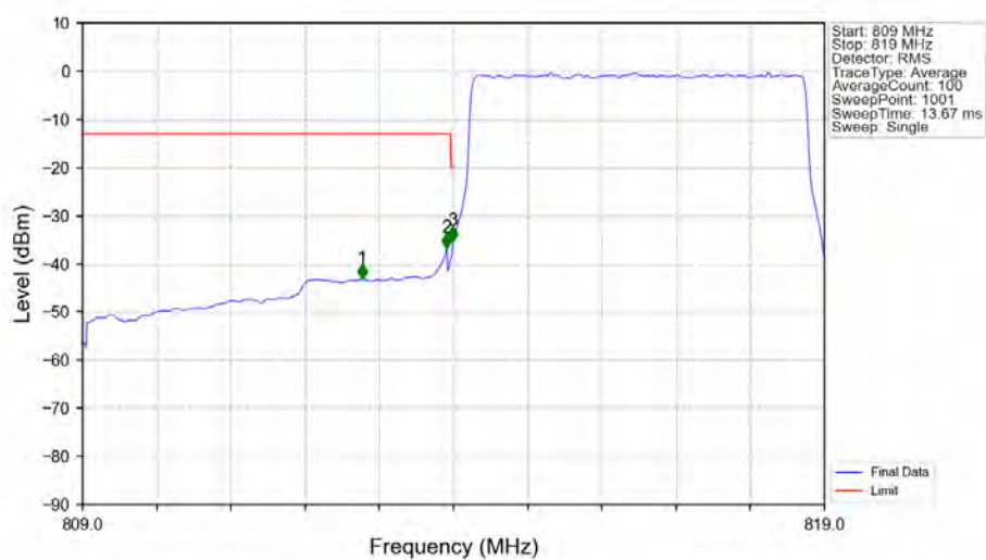
Band26a 5MHz 256QAM LCH 816.5MHz RB 25 0 NTNV
