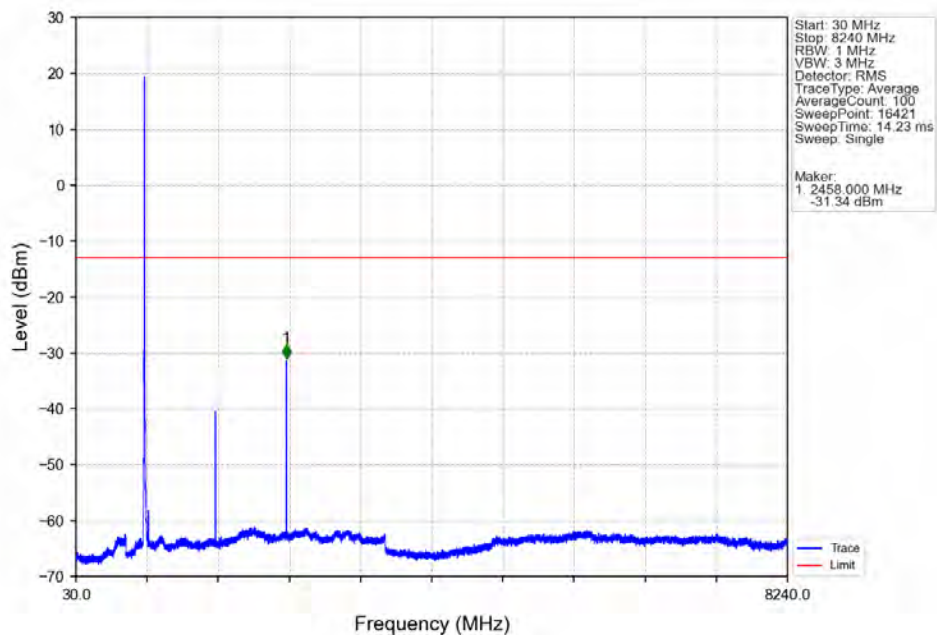
Band26a 5MHz 64QAM HCH 821.5MHz RB 1 24 NTNV
