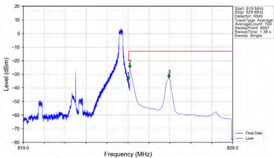
Band26a 5MHz 256QAM HCH 821.5MHz RB 1 24 NTNV
