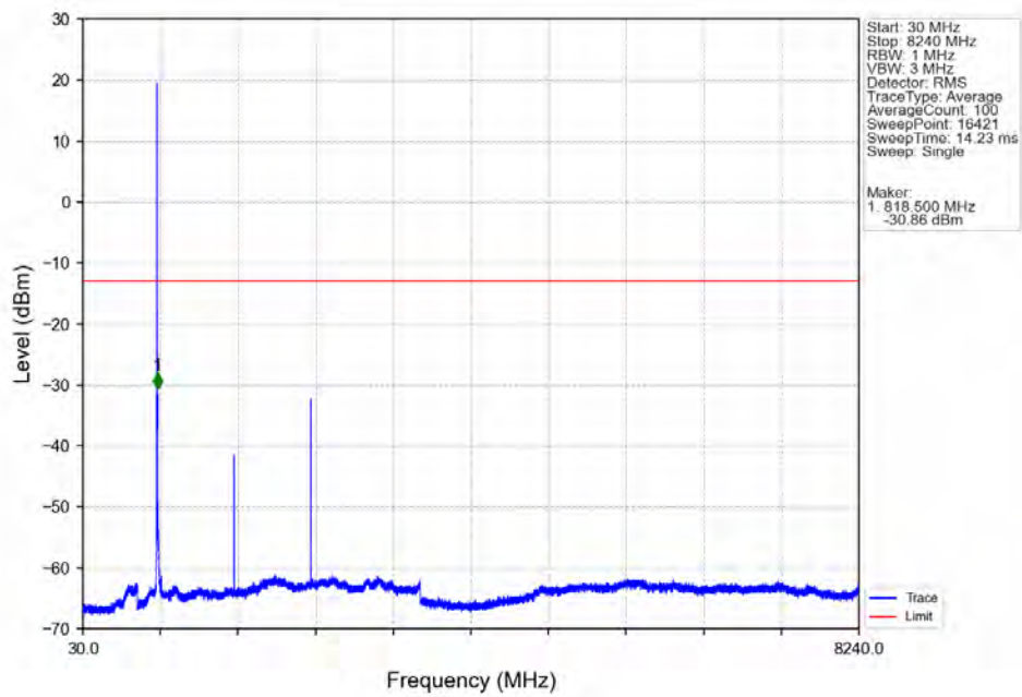
Band26a 1.4MHz 64QAM LCH 814.7MHz RB 1 0 NTNV
