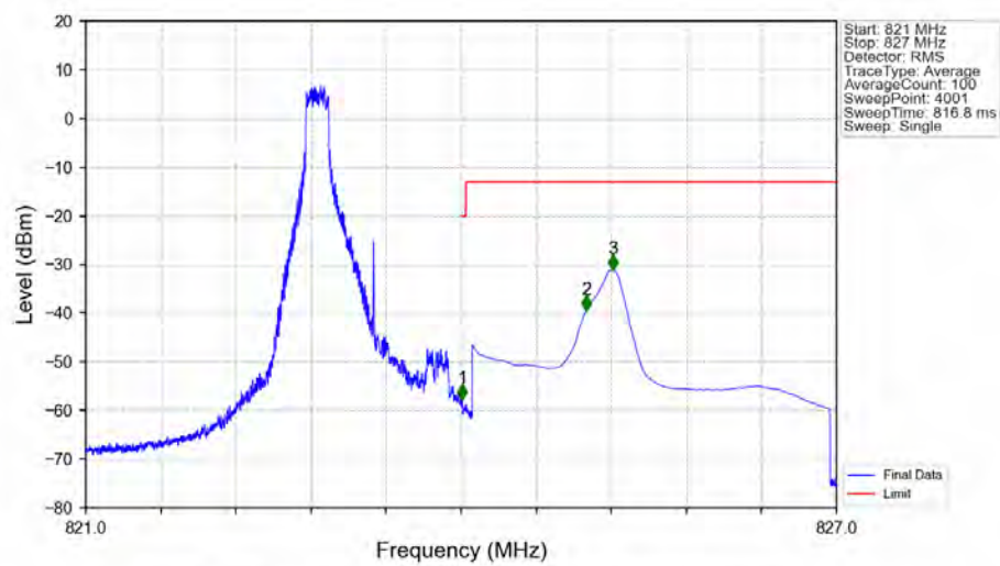
Band26a 1.4MHz QPSK HCH 823.3MHz RB 1 5 NTV
