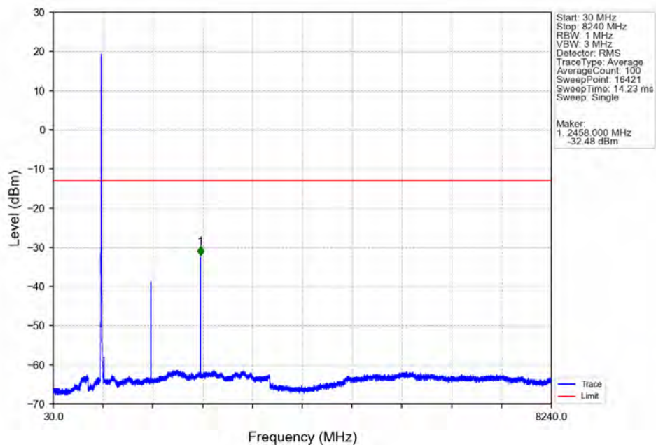
Band26a 5MHz QPSK HCH 821.5MHz RB 1 24 NTV
