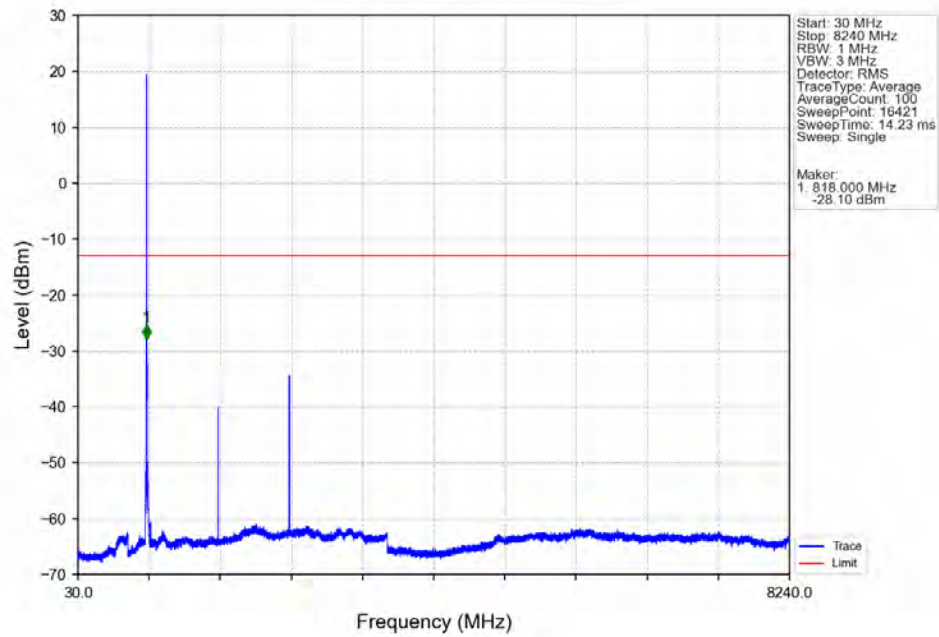
Band26a 1.4MHz QPSK HCH 823.3MHz RB 1 5 NTV
