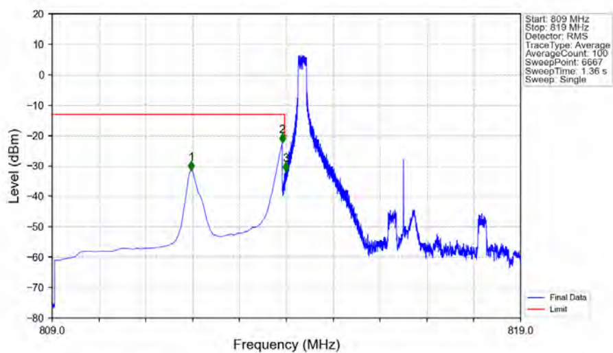
Band26a 5MHz 64QAM LCH 816.5MHz RB 1 0 NTNV
