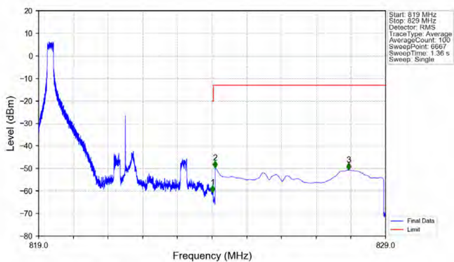
Band26a 5MHz QPSK HCH 821.5MHz RB 1 24 NTV
