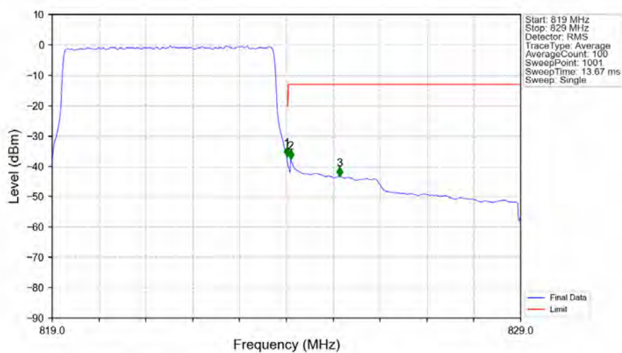
Band26a 5MHz 256QAM HCH 821.5MHz RB 25 0 NTNV
