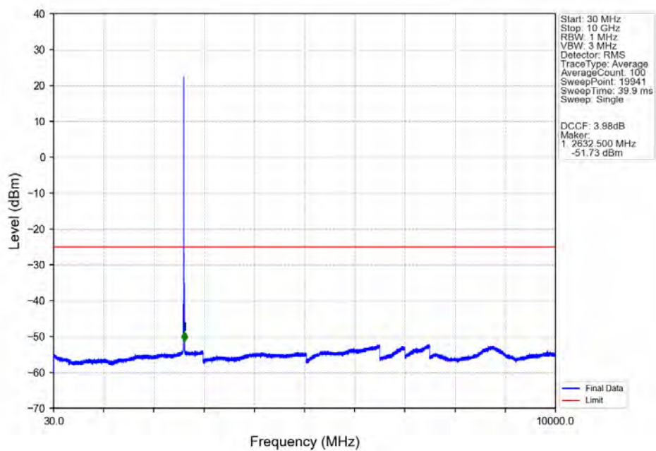
Band38 5MHz 16QAM HCH 2617.5MHz RB 1 0 NTV
