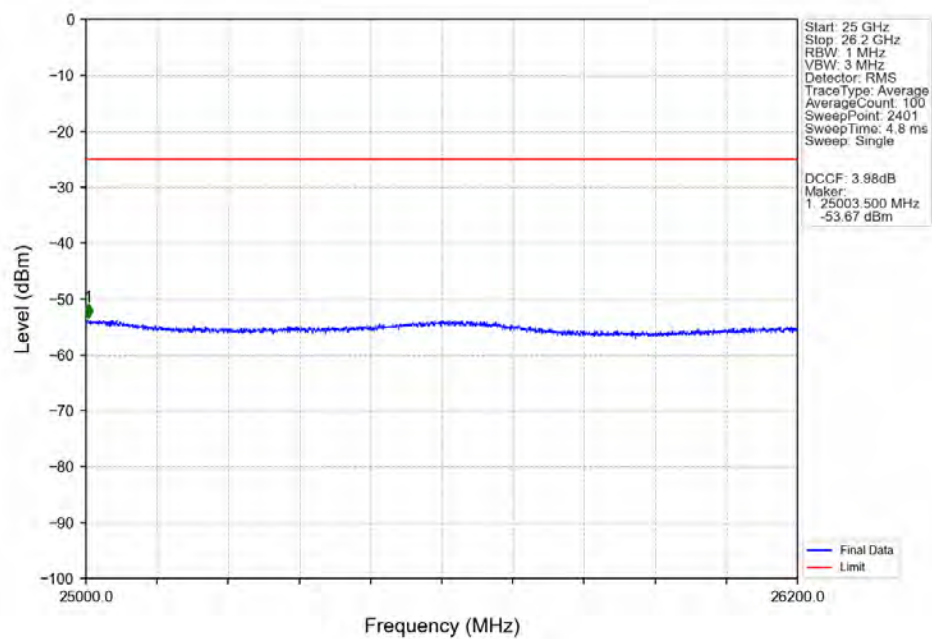
Band38 5MHz 16QAM HCH 2617.5MHz RB 1 0 NTNV
