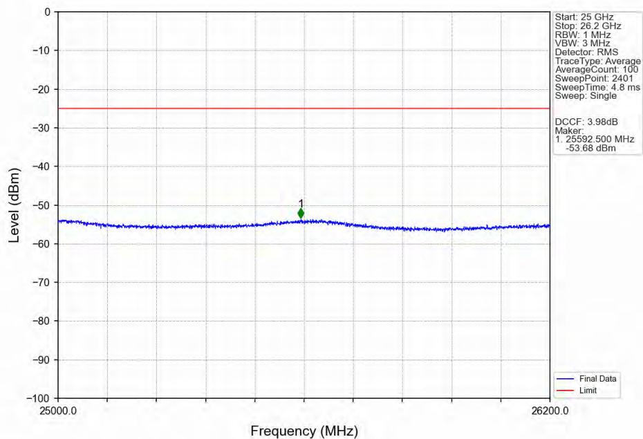
Band38 5MHz 16QAM HCH 2617.5MHz RB 1 0 NTV
