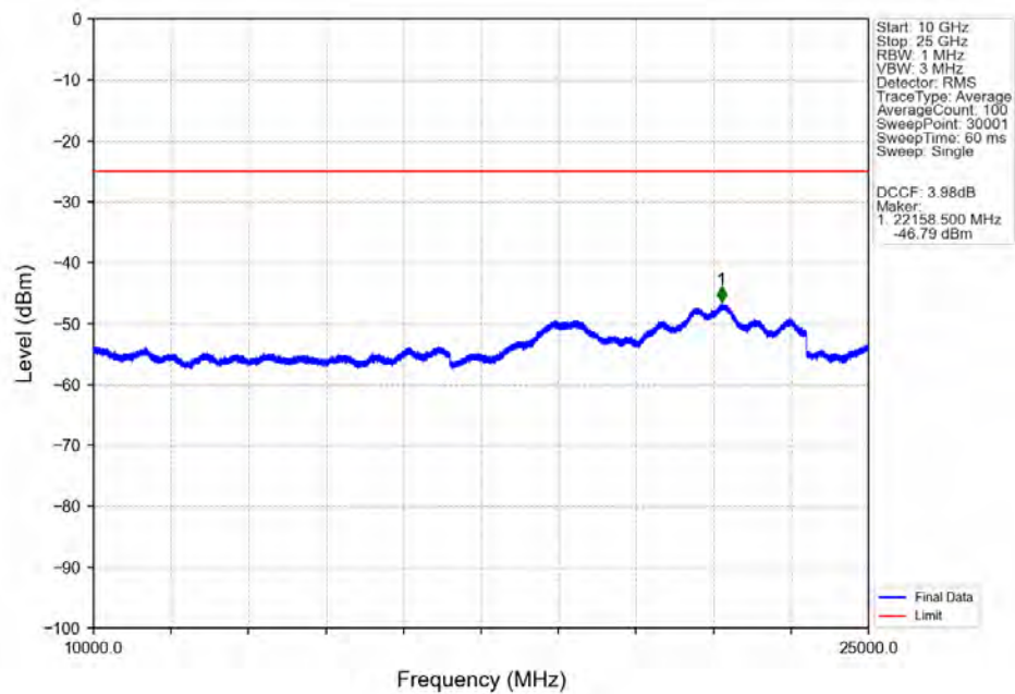
Band38 5MHz 16QAM HCH 2617.5MHz RB 1 0 NTNV
