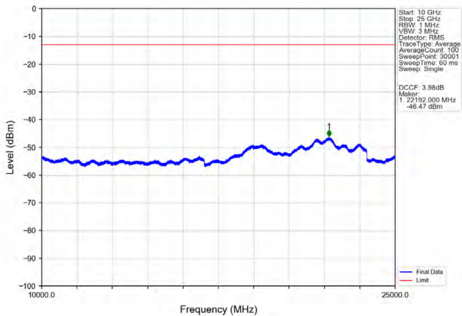
Band42a 5MHz 64QAM MCH 3500MHz RB 1 0 NTNV
