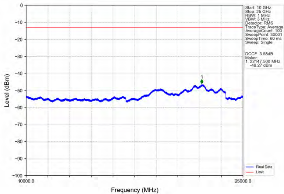
Band42a 5MHz 16QAM HCH 3547.5MHz RB 1 0 NTNV
