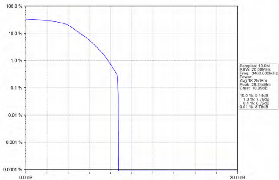
Band42a_20MHz_QPSK_LCH_3460MHz_RB_100_0_NTNV
