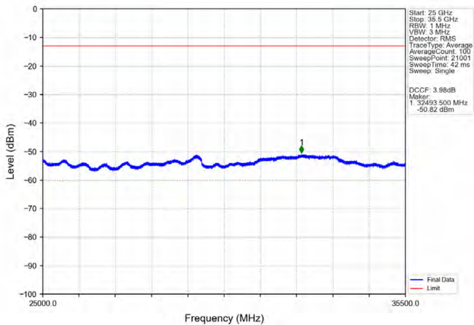
Band42a 5MHz 16QAM HCH 3547.5MHz RB 1 0 NTNV
