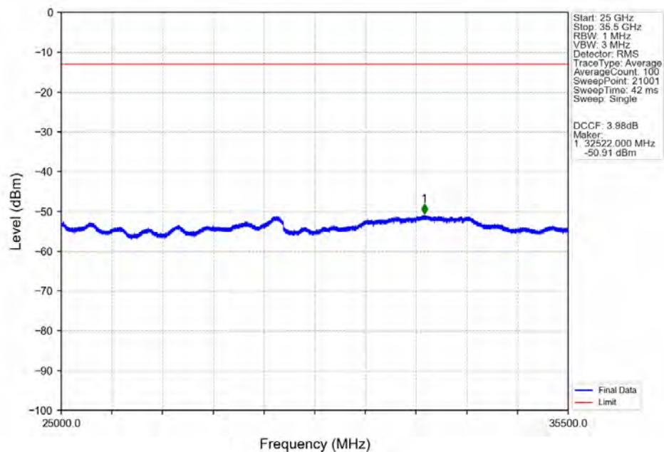
Band42a 5MHz 64QAM HCH 3547.5MHz RB 1 24 NTNV
