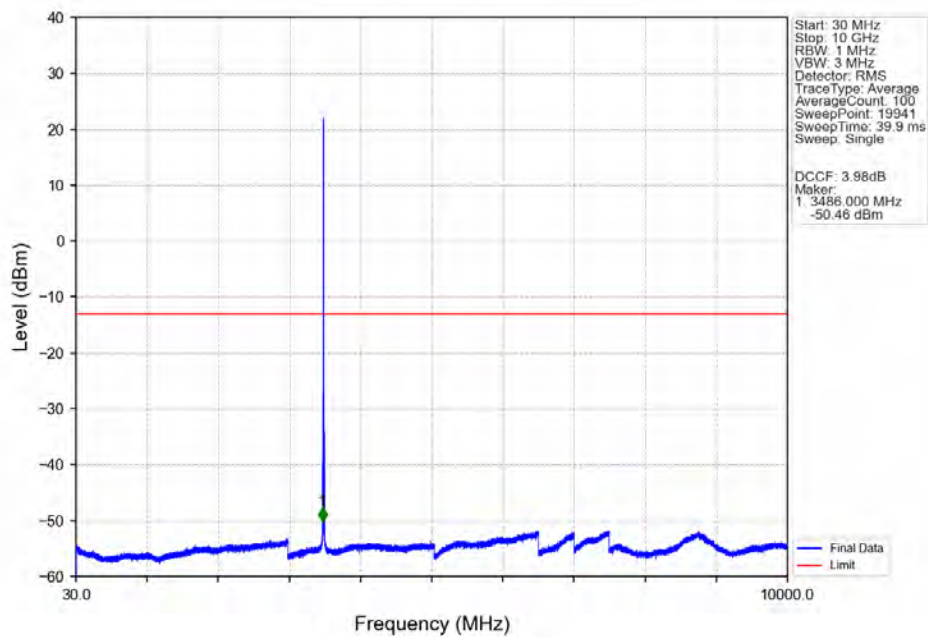
Band42a 5MHz 16QAM MCH 3500MHz RB 1 0 NTNV
