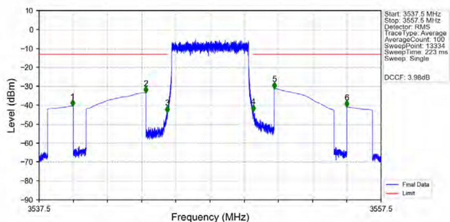
Band42a 5MHz 64QAM HCH 3547.5MHz RB 1 24 NTNV
