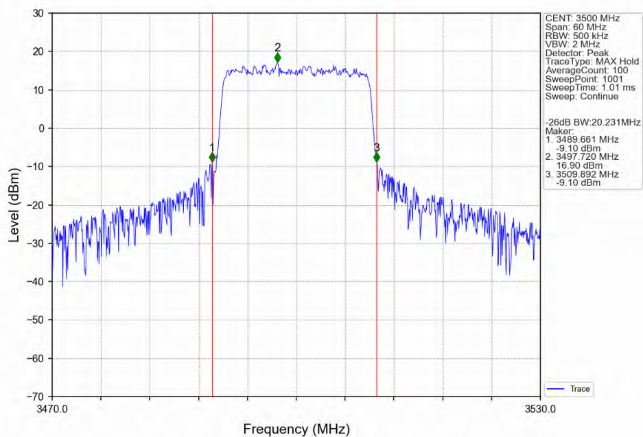
Band42a 20MHz 64QAM MCH 3500MHz RB 100 0 NTN
