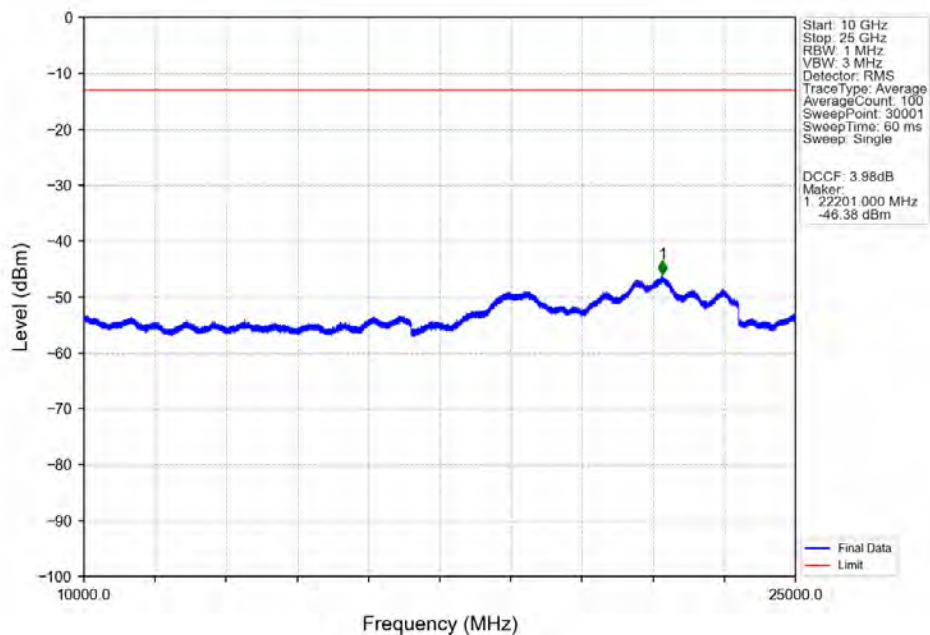
Band42a 5MHz QPSK LCH 3452.5MHz RB 1 0 NTNV
