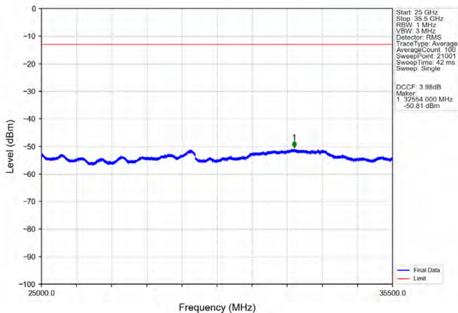
Band42a 5MHz QPSK HCH 3547.5MHz RB 1 24 NTNV
