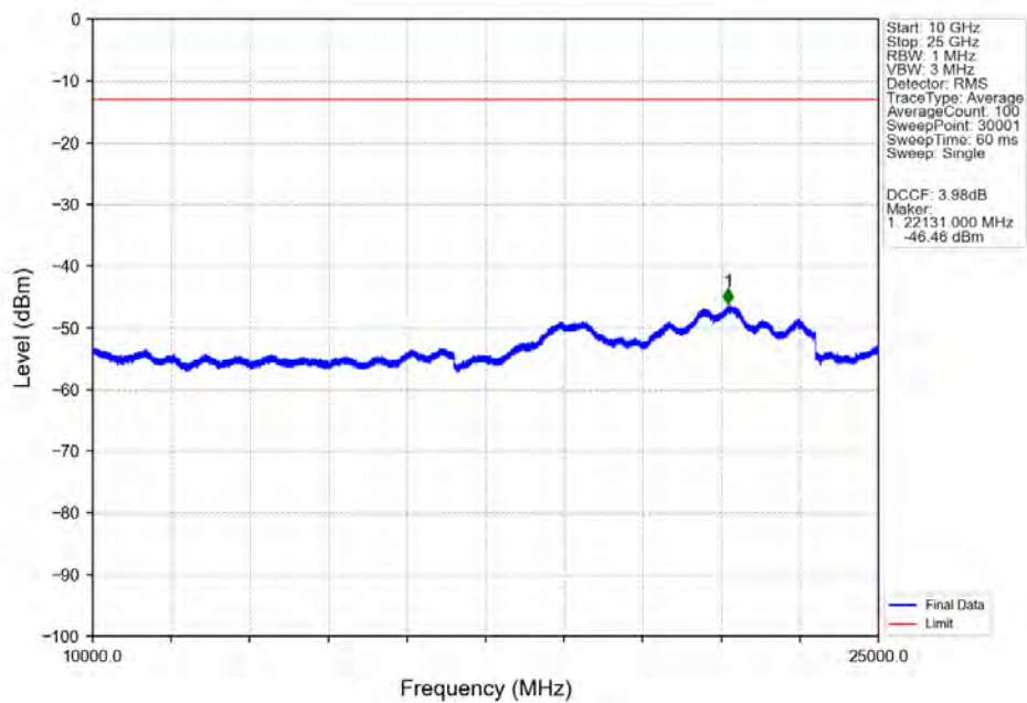
Band42a 5MHz QPSK MCH 3500MHz RB 1 0 NTNV
