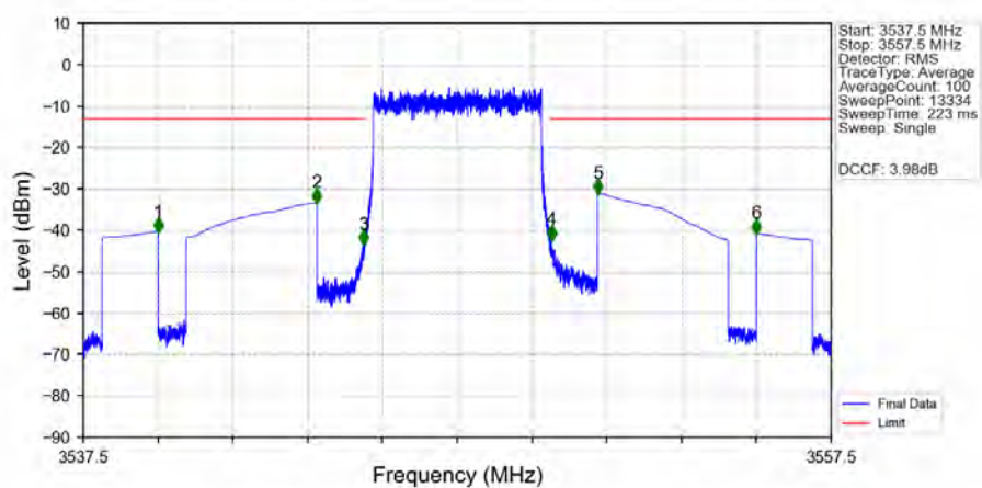
Band42a 5MHz QPSK HCH 3547.5MHz RB 1 24 NTNV
