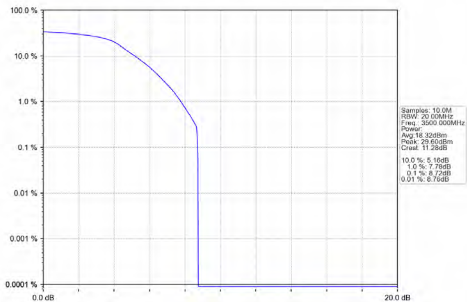
Band42a_20MHz_QPSK_MCH_3500MHz_RB_100_0_NTNV
