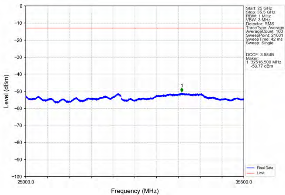
Band42a 5MHz QPSK LCH 3452.5MHz RB 1 0 NTNV
