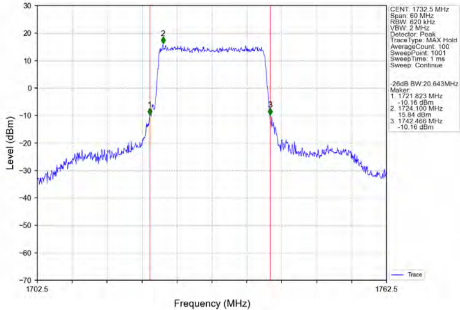
Band4_20MHz_QPSK_MCH_1732.5MHz_RB_100_0_NTNV
