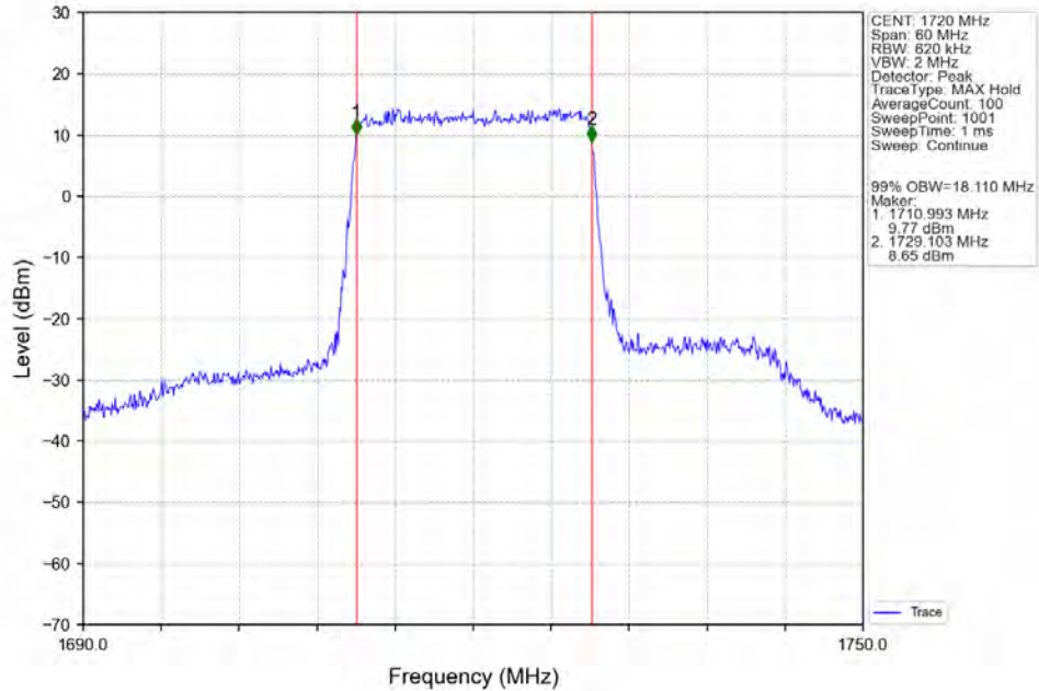
Band4_20MHz_256QAM_LCH_1720MHz_RB_100_0_NTNV
