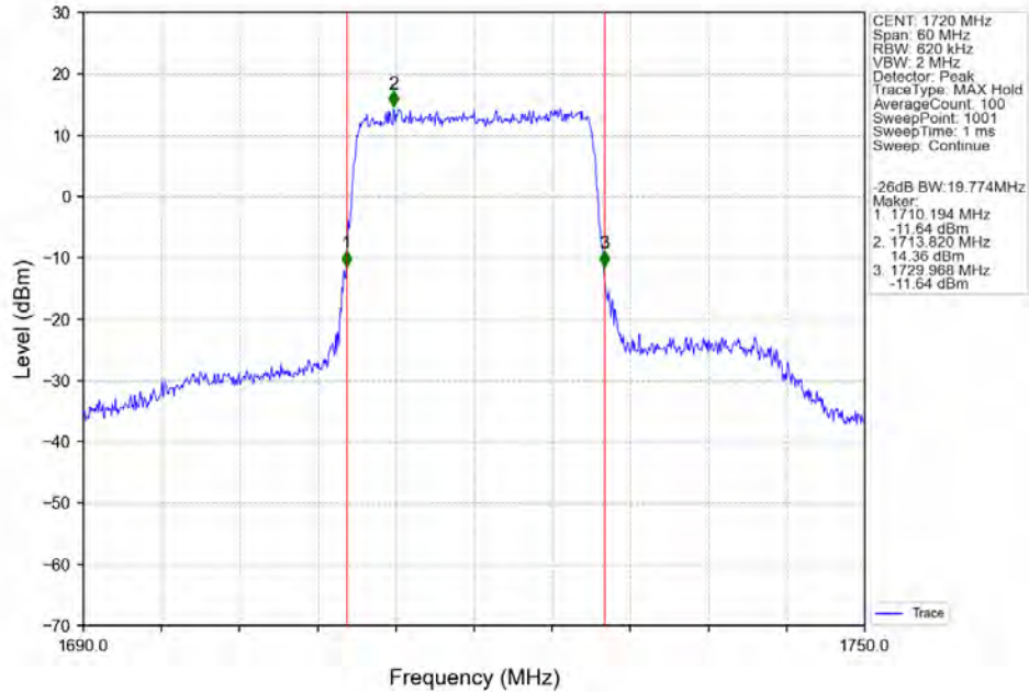
Band4_20MHz_256QAM_LCH_1720MHz_RB_100_0_NTNV
