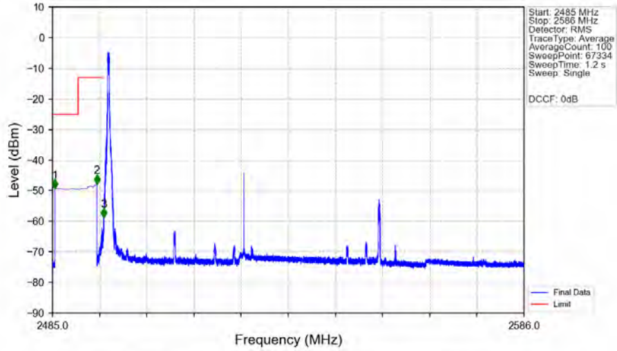
n41_30kHz_SISO_NTNV_60MHz_CP-OFDM_QPSK_2526MHz_Edge_1RB_Left_Ant1
