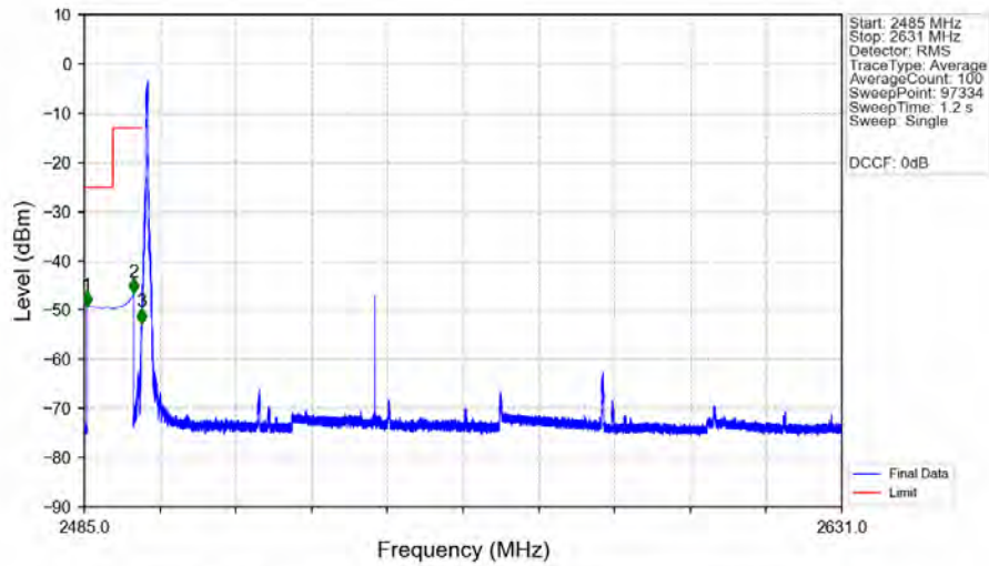
n41_30kHz_SISO_NTNV_90MHz_DFT-s-OFDM PI/2 BPSK_2541MHz_Edge_1RB_Left_Ant1
