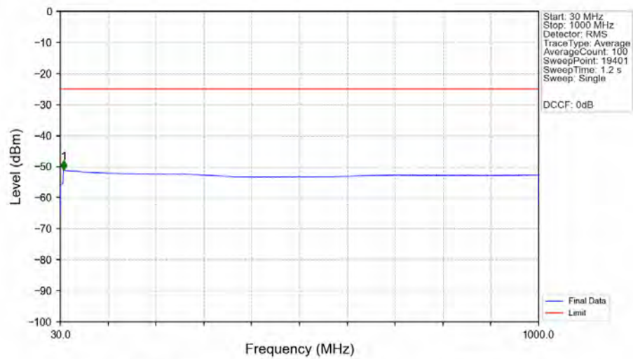
n41_30kHz_SISO_NTNV_60MHz_CP-OFDM_QPSK_2526MHz_Edge_1RB_Left_Ant1
