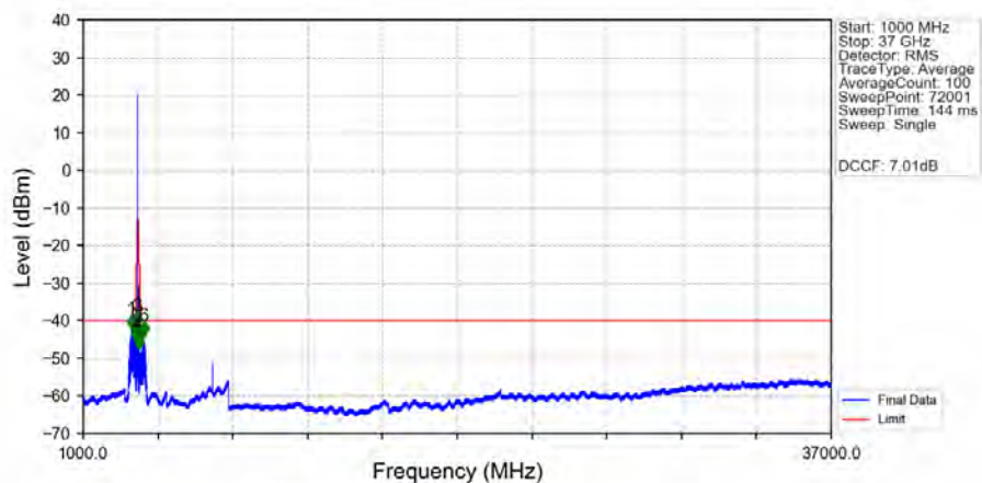
n48_30kHz_SISO_NTNV_20MHz_DFT-s-OFDM PI/2 BPSK_3624.99MHz_Edge_1RB_Left_Ant1
