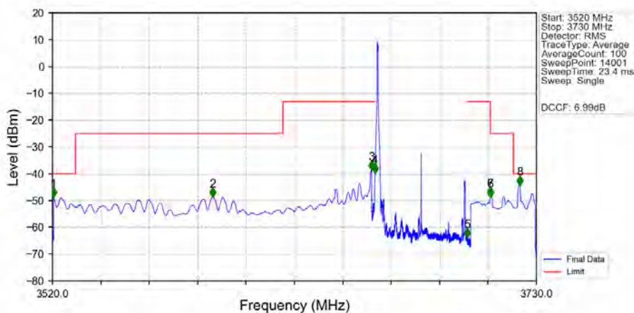
n48_30kHz_SISO_NTNV_40MHz_CP-OFDM_QPSK_3679.98MHz_Edge_1RB_Left_Ant1
