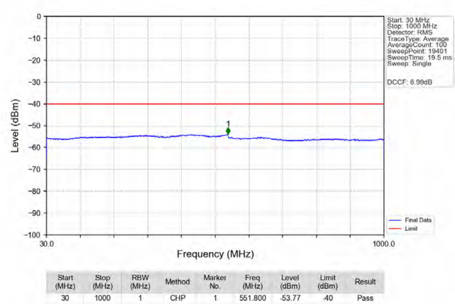
n48_30kHz_SISO_NTNV_40MHz_CP-OFDM_QPSK_3570MHz_Edge_1RB_Left_Ant1
