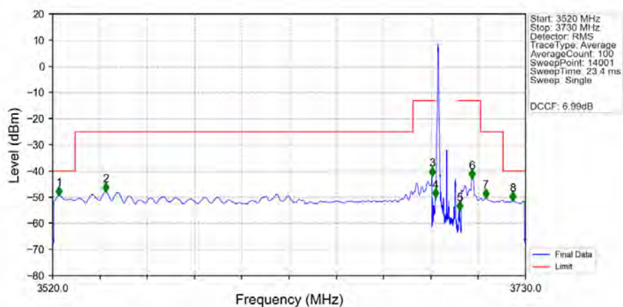
n48_30kHz_MIMO_NTNV_10MHz_DFT-s-OFDM_PI/2_BPSK_3694.98MHz_Inner_1RB_Left_Ant2
