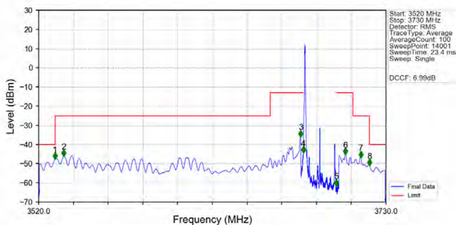
n48_30kHz_SISO_NTNV_20MHz_DFT-s-OFDM PI/2 BPSK_3690MHz_Edge_1RB_Left_Ant1
