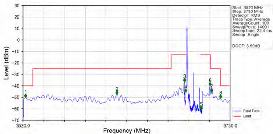
n48_30kHz_SISO_NTNV_15MHz_CP-OFDM_QPSK_3692.49MHz_Inner_1RB_Left_Ant1
