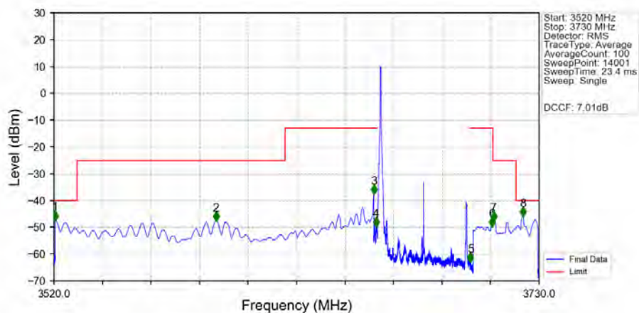
n48_30kHz_SISO_NTNV_40MHz_CP-OFDM_QPSK_3679.98MHz_Inner_1RB_Left_Ant1
