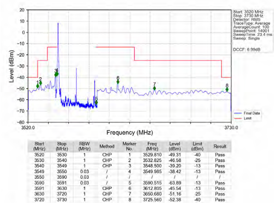
n48_30kHz_SISO_NTNV_40MHz_CP-OFDM_QPSK_3570MHz_Edge_1RB_Left_Ant1
