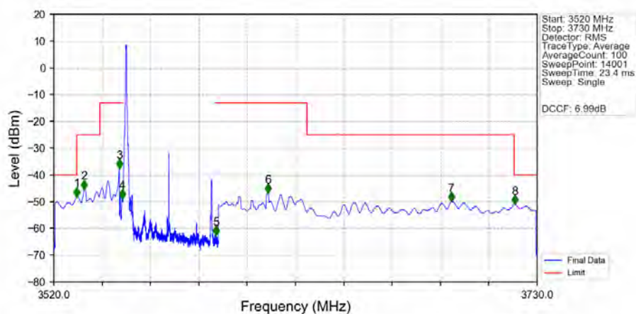
n48_30kHz_SISO_NTNV_40MHz_CP-OFDM_QPSK_3570MHz_Inner_1RB_Left_Ant1
