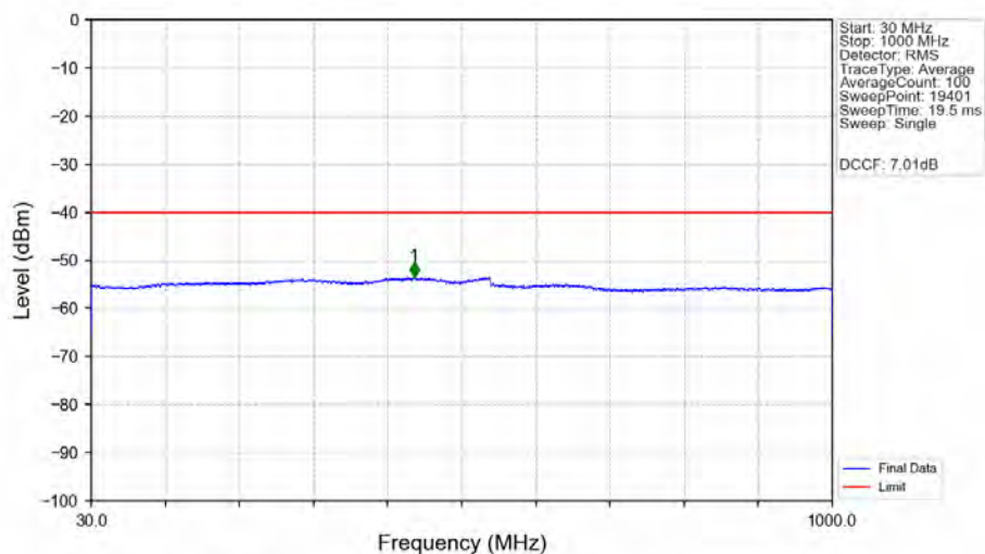
n48_30kHz_SISO_NTNV_20MHz_CP-OFDM_QPSK_3624.99MHz_Edge_1RB_Left_Ant1
