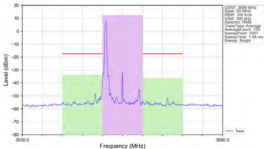
n48_30kHz_SISO_NTNV_10MHz_CP-OFDM 64 QAM 3555MHz_Edge_1RB_Left_Ant1
