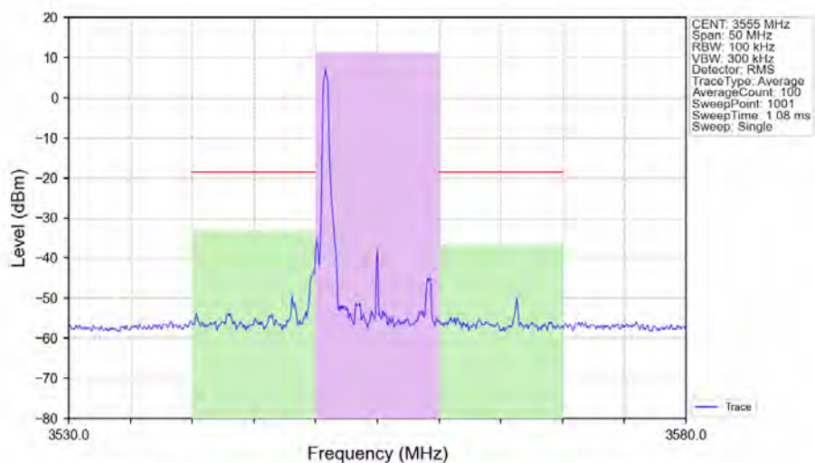
n48_30kHz_SISO_NTNV_10MHz_DFT-s-OFDM PI/2 BPSK_3555MHz_Edge_1RB_Left_Ant1
