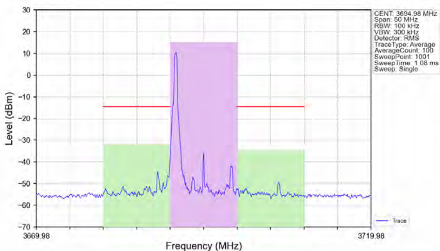
n48_30kHz_SISO_NTNV_10MHz_DFT-s-OFDM_PI/2_BPSK_3694.98MHz_Edge_1RB_Left_Ant1
