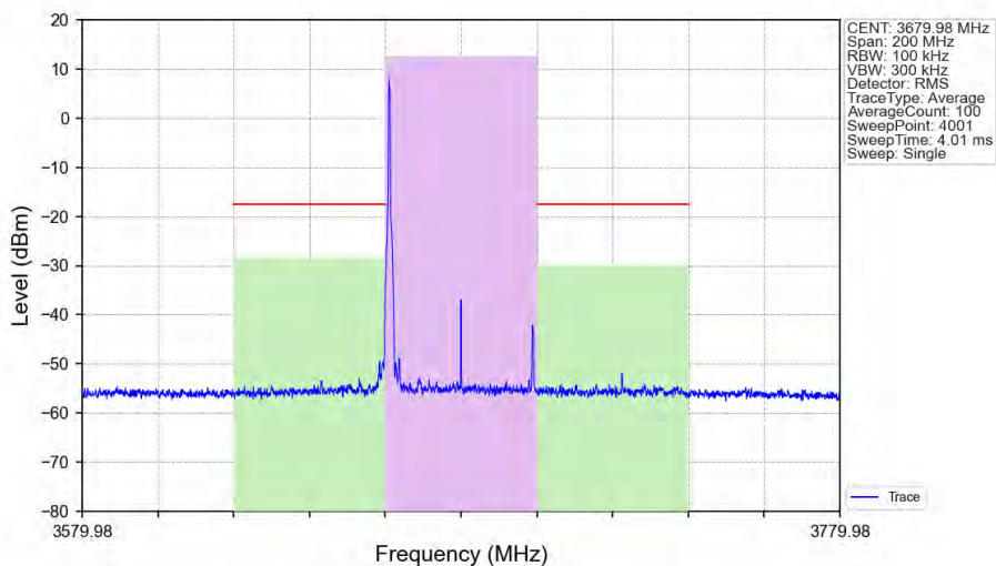
n48_30kHz_SISO_NTNV_40MHz_CP-OFDM_QPSK_3679.98MHz_Edge_1RB_Left_Ant1
