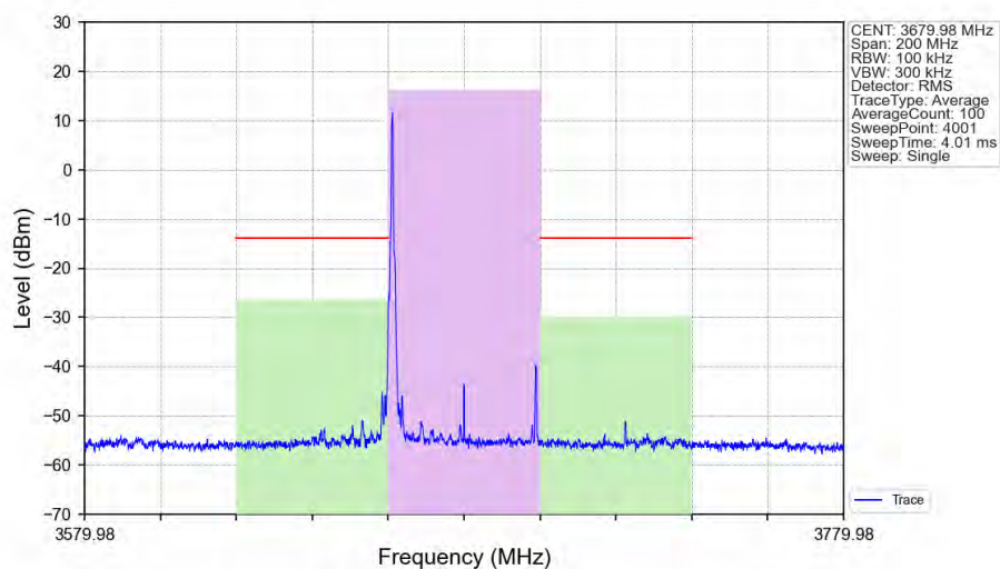
n48_30kHz_SISO_NTNV_40MHz_DFT-s-OFDM_PI/2_BPSK_3679.98MHz_Edge_1RB_Left_Ant1
