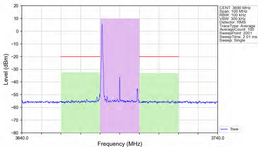
n48_30kHz_SISO_NTNV_20MHz_CP-OFDM 256 QAM 3690MHz_Edge_1RB_Left_Ant1
