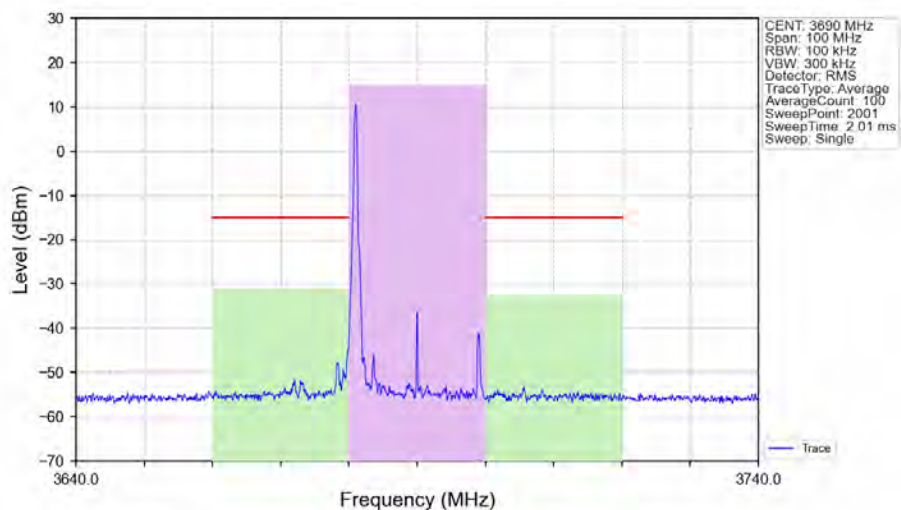
n48_30kHz_SISO_NTNV_20MHz_DFT-s-OFDM_QPSK_3690MHz_Edge_1RB_Left_Ant1
