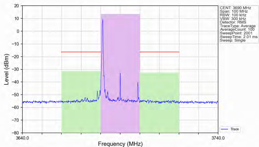
n48_30kHz_SISO_NTNV_20MHz_DFT-s-OFDM_16_QAM_3690MHz_Edge_1RB_Left_Ant1
