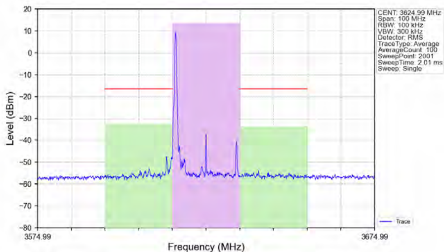
n48_30kHz_SISO_NTNV_20MHz_DFT-s-OFDM PI/2 BPSK_3624.99MHz_Edge_1RB_Left_Ant1
