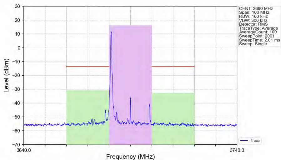
n48_30kHz_SISO_NTNV_20MHz_DFT-s-OFDM_PI/2_BPSK_3690MHz_Edge_1RB_Left_Ant1
