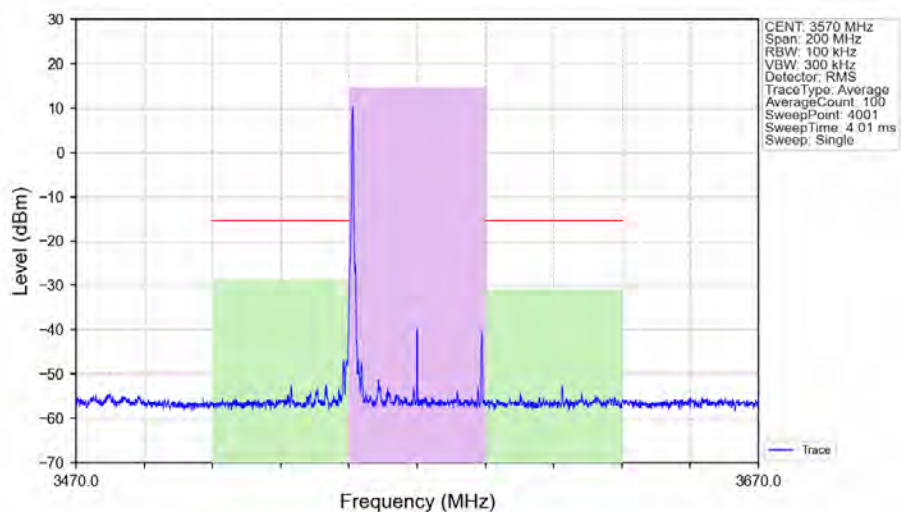
n48_30kHz_SISO_NTNV_40MHz_DFT-s-OFDM PI/2 BPSK_3570MHz_Edge_1RB_Left_Ant1
