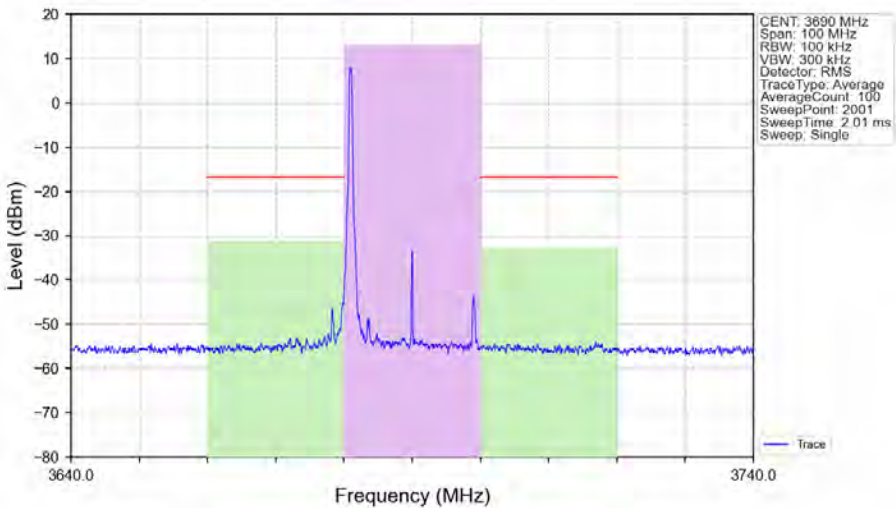
n48_30kHz_SISO_NTNV_20MHz_CP-OFDM_QPSK_3690MHz_Edge_1RB_Left_Ant1
