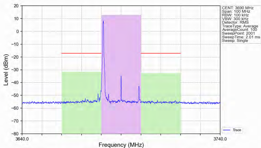
n48_30kHz_SISO_NTNV_20MHz_CP-OFDM_16_QAM_3690MHz_Edge_1RB_Left_Ant1
