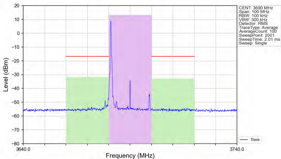
n48_30kHz_SISO_NTNV_20MHz_CP-OFDM 64 QAM 3690MHz_Edge_1RB_Left_Ant1
