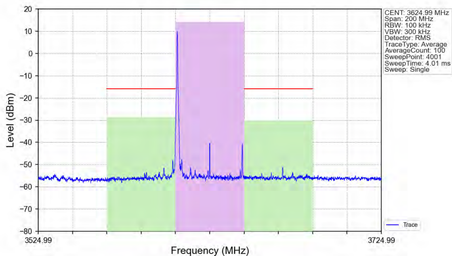
n48_30kHz_SISO_NTNV_40MHz_DFT-s-OFDM PI/2 BPSK_3624.99MHz_Edge_1RB_Left_Ant1
