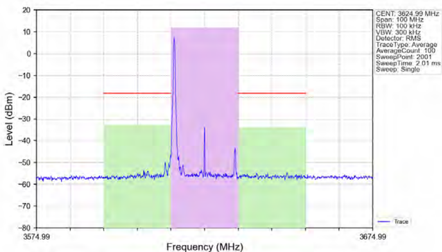
n48_30kHz_SISO_NTNV_20MHz_CP-OFDM_QPSK_3624.99MHz_Edge_1RB_Left_Ant1
