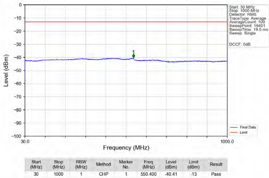
n66 15kHz MIMO NTNv 20MHz CP-OFDM QPSK 1770MHz Edge 1RB Right Ant1
