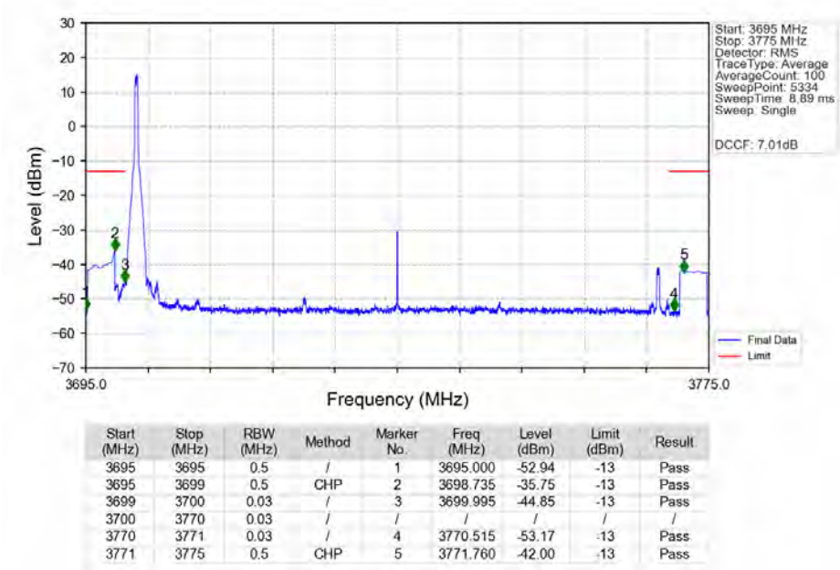
n77a_30kHz_SISO_NTNV_70MHz_CP-OFDM_QPSK_3735MHz_Inner_1RB_Left_Ant1
