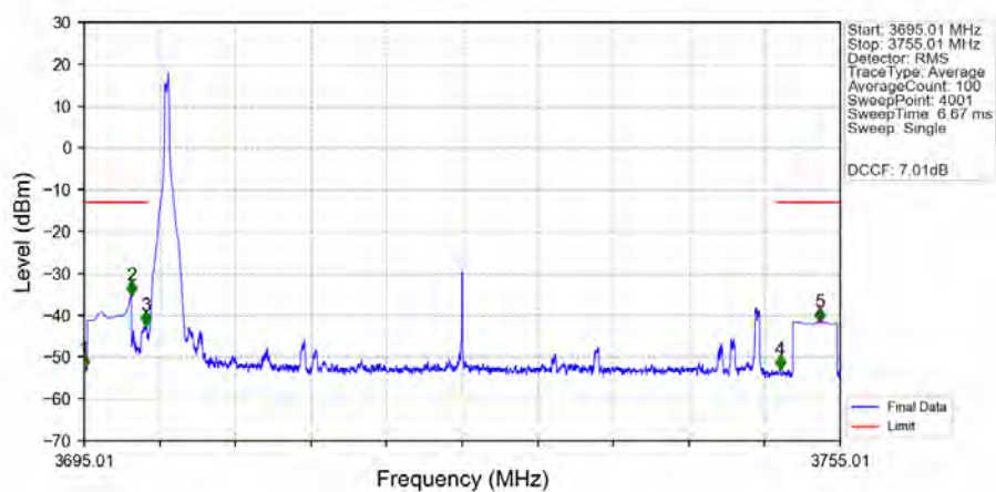
n77a_30kHz_SISO_NTNV_50MHz_DFT-s-OFDM_PI/2_BPSK_3725.01MHz_Inner_1RB_Left_Ant1
