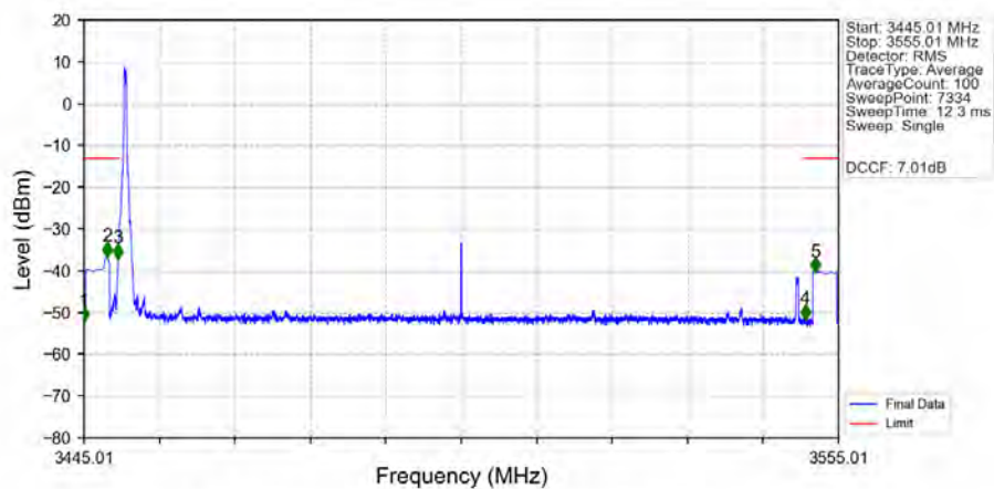
n78e 30kHz MIMO NTNV 100MHz CP-OFDM QPSK 3500.01MHz Edge 1RB Left Ant1
