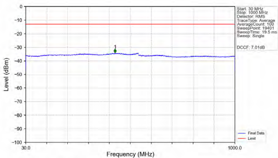
n78e 30kHz MIMO NTV 100MHz CP-OFDM QPSK 3500.01MHz Edge 1RB Left Ant1
